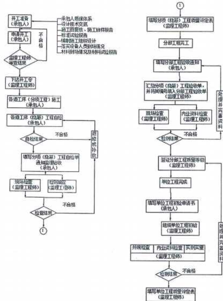
工程质量控制程序流程图
