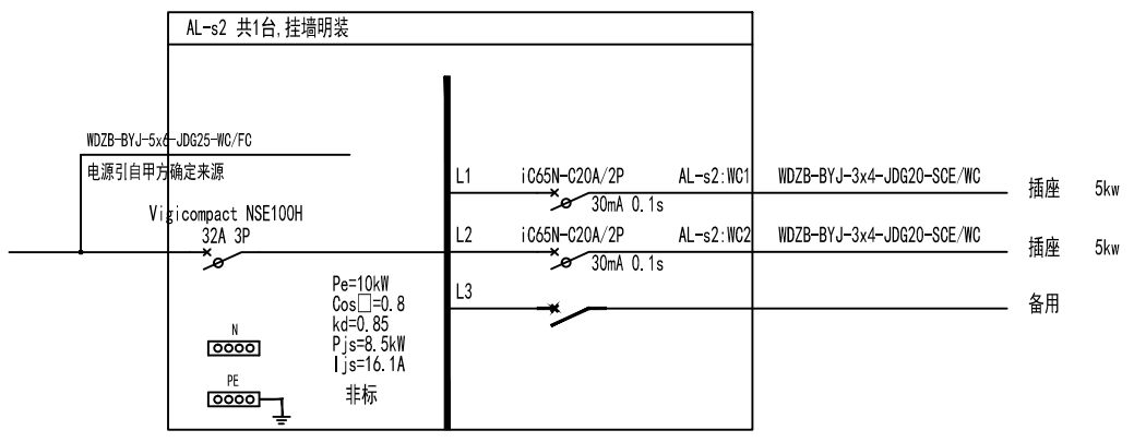
AL-s2配电箱
