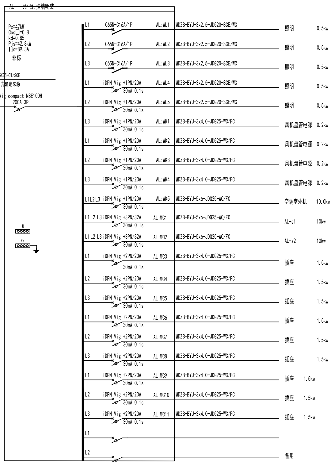
AL配电箱
