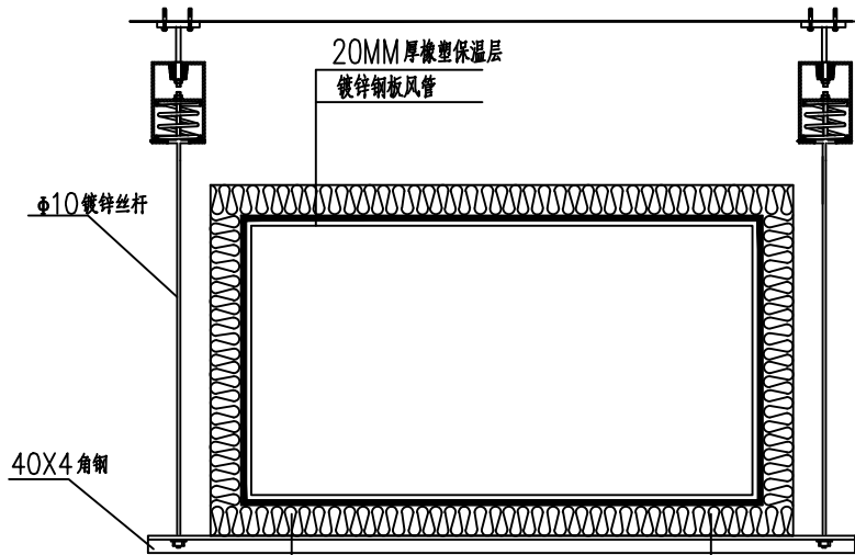
风管安装示意图
