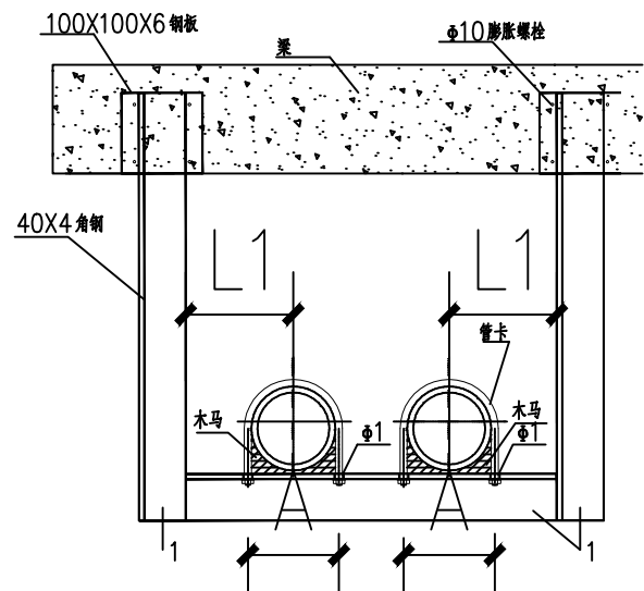
水管支架图
