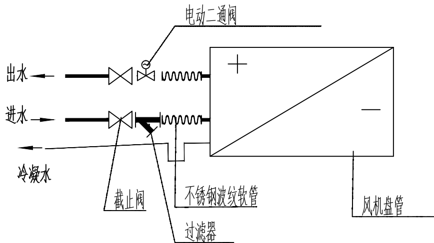
风机盘管接管示意图
