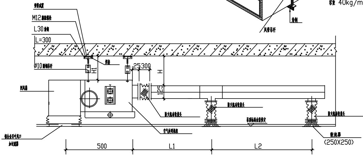
风机盘管接风管安装大样(多出口)
