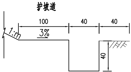
排水沟 I
