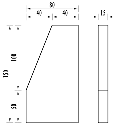
肋板大样图
