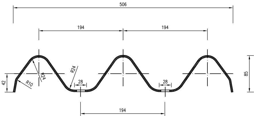
N端—II—断面图
