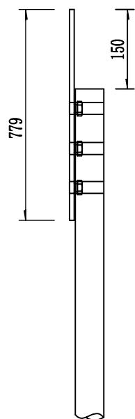
标志板侧面图
