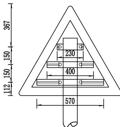
标志板背面图
