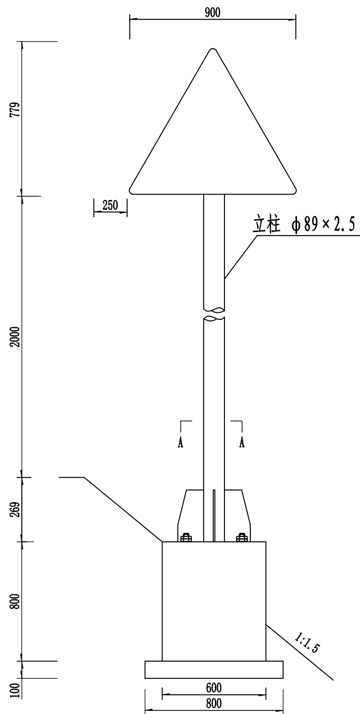
标志牌立面图
