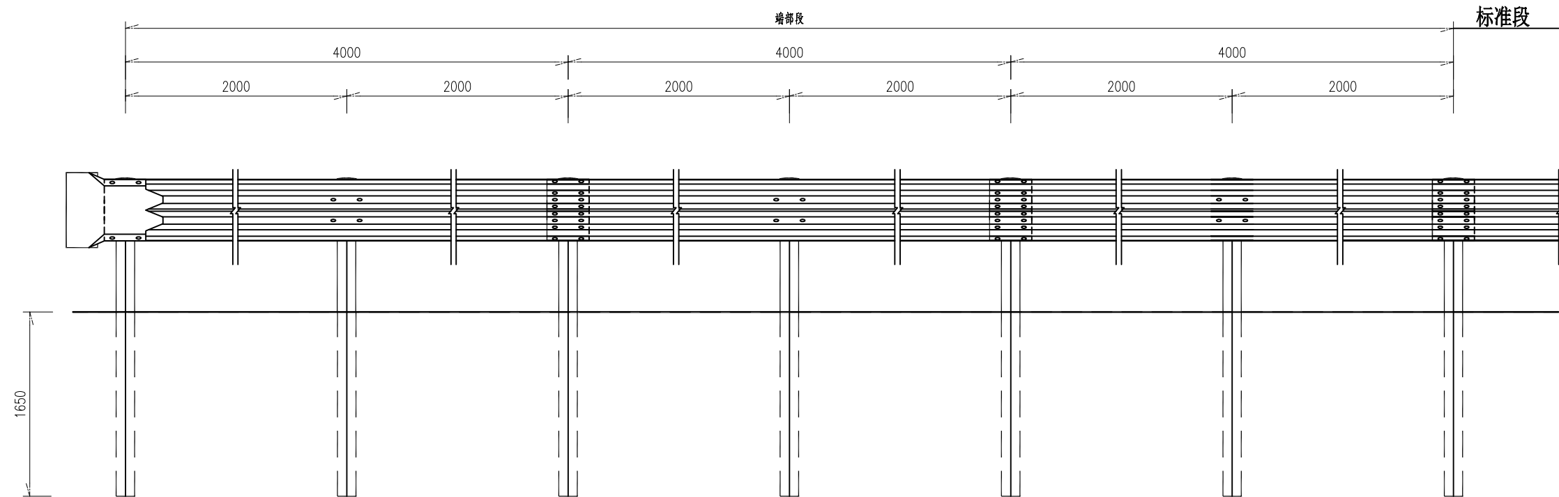
下游端头立面图
