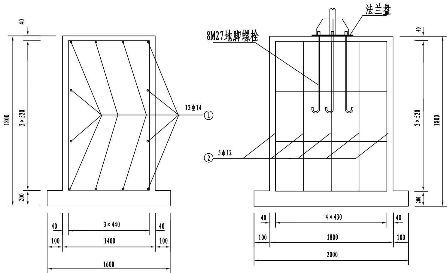
基础立面图
