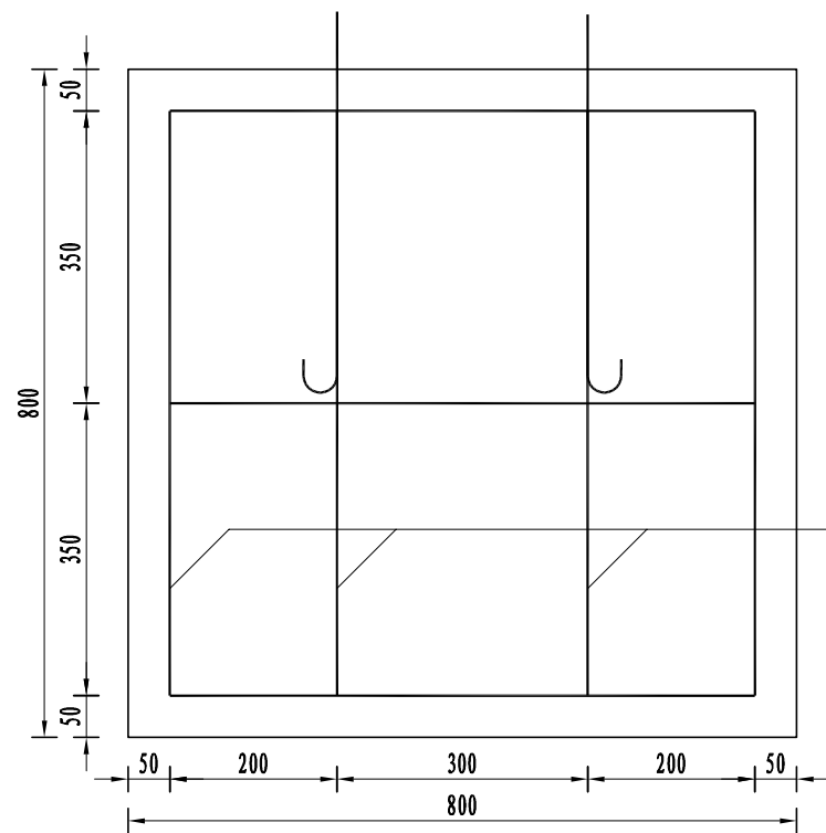
侧面图 1:10
