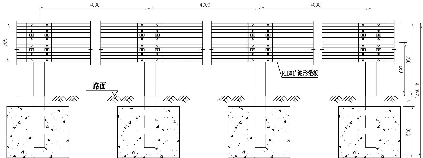
立面图 1:25 Gr-A-4C
