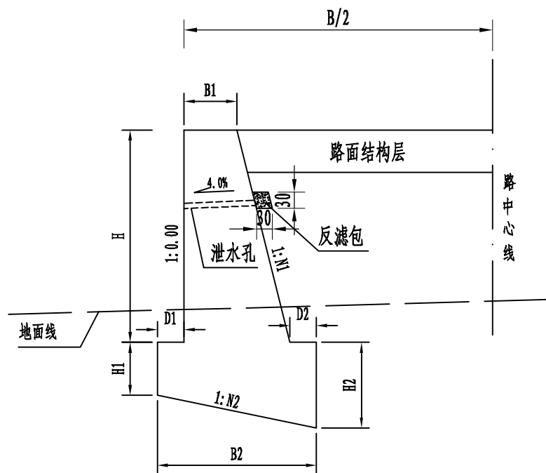
路肩式挡土墙图示
