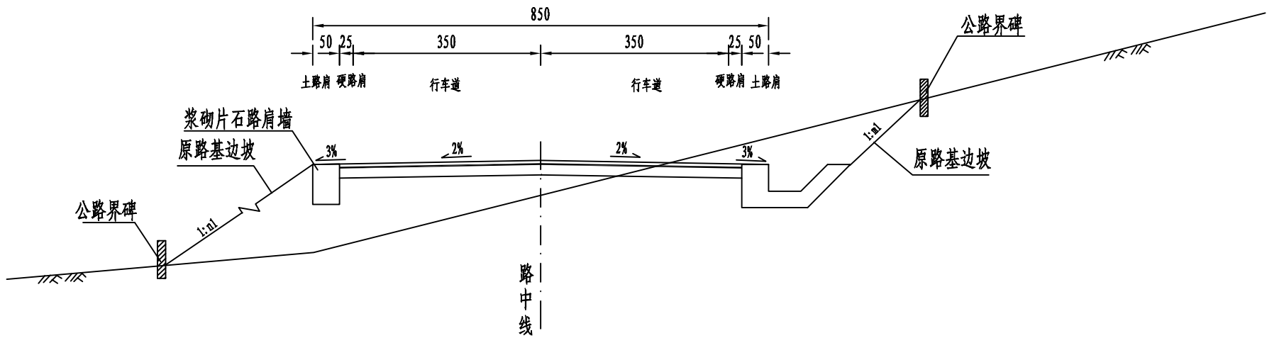
路基标准横断面图 1:100
