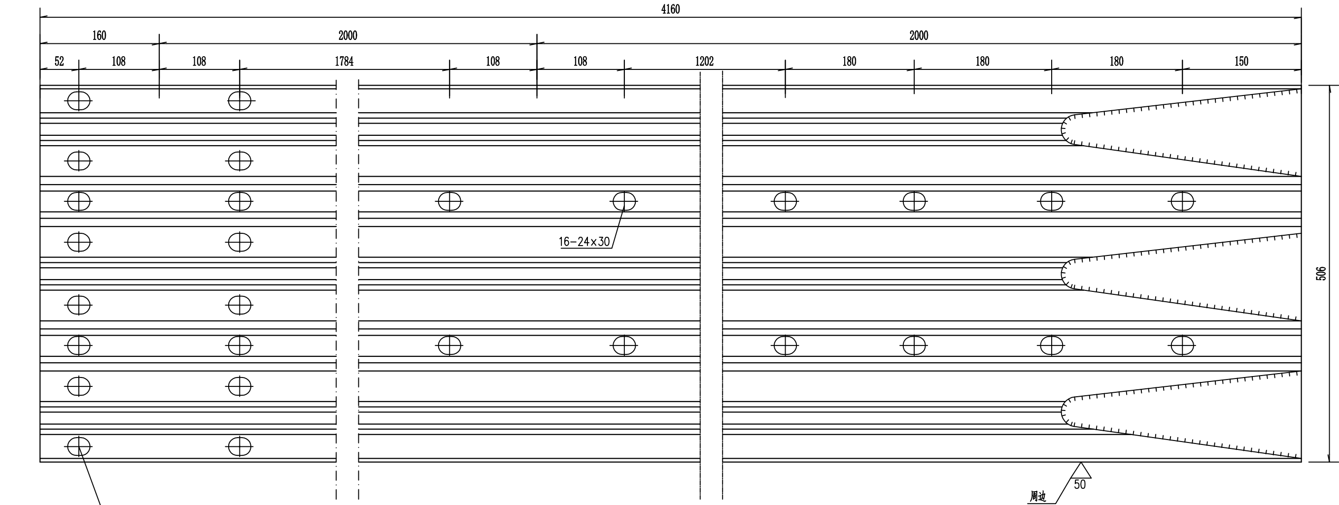
RTB04'平面图
