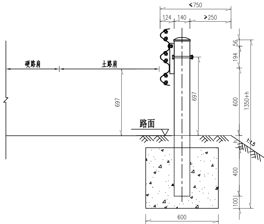
侧面图 1:20 Gr-A-4C
