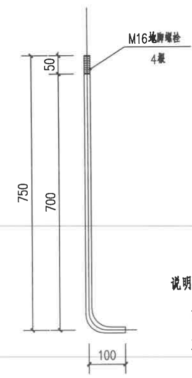
地脚螺栓大样图 1:10
