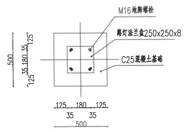
路灯基础平面做法 1:20
