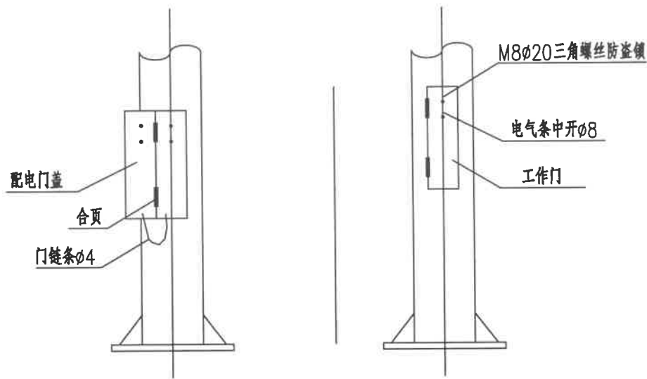
工作门 1:10
