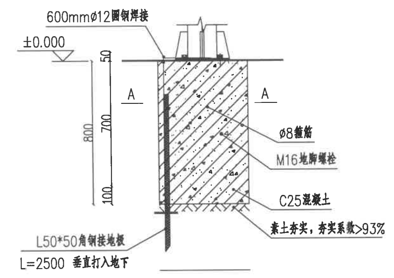
路灯基础立面做法 1:20
