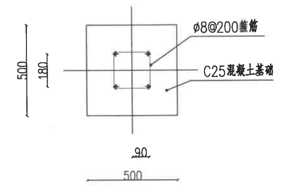
A-A断面图 1:20
