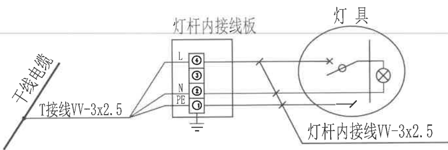
路灯电气接线示意图 1:10
