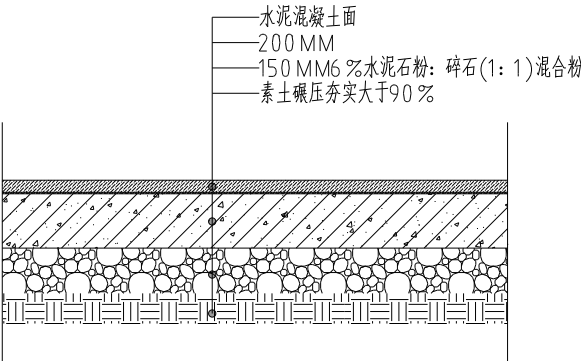
基地道路详图
