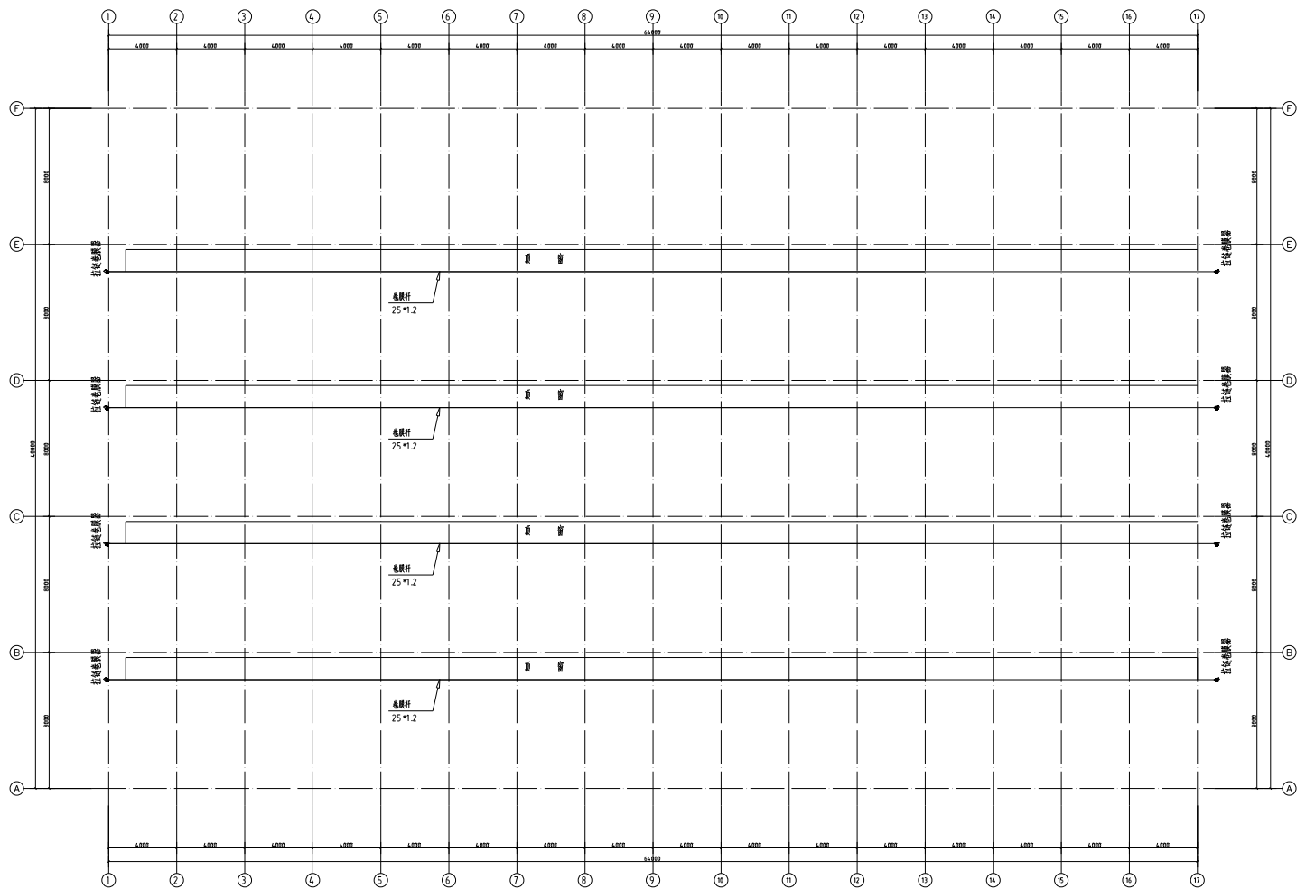
2 屋面骨架布置图
