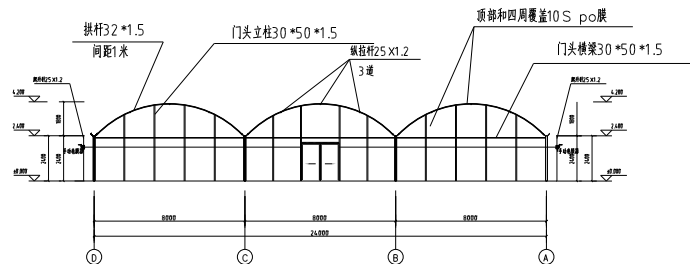
1D~A立面图
