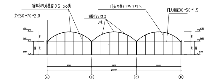
1A~D立面图
