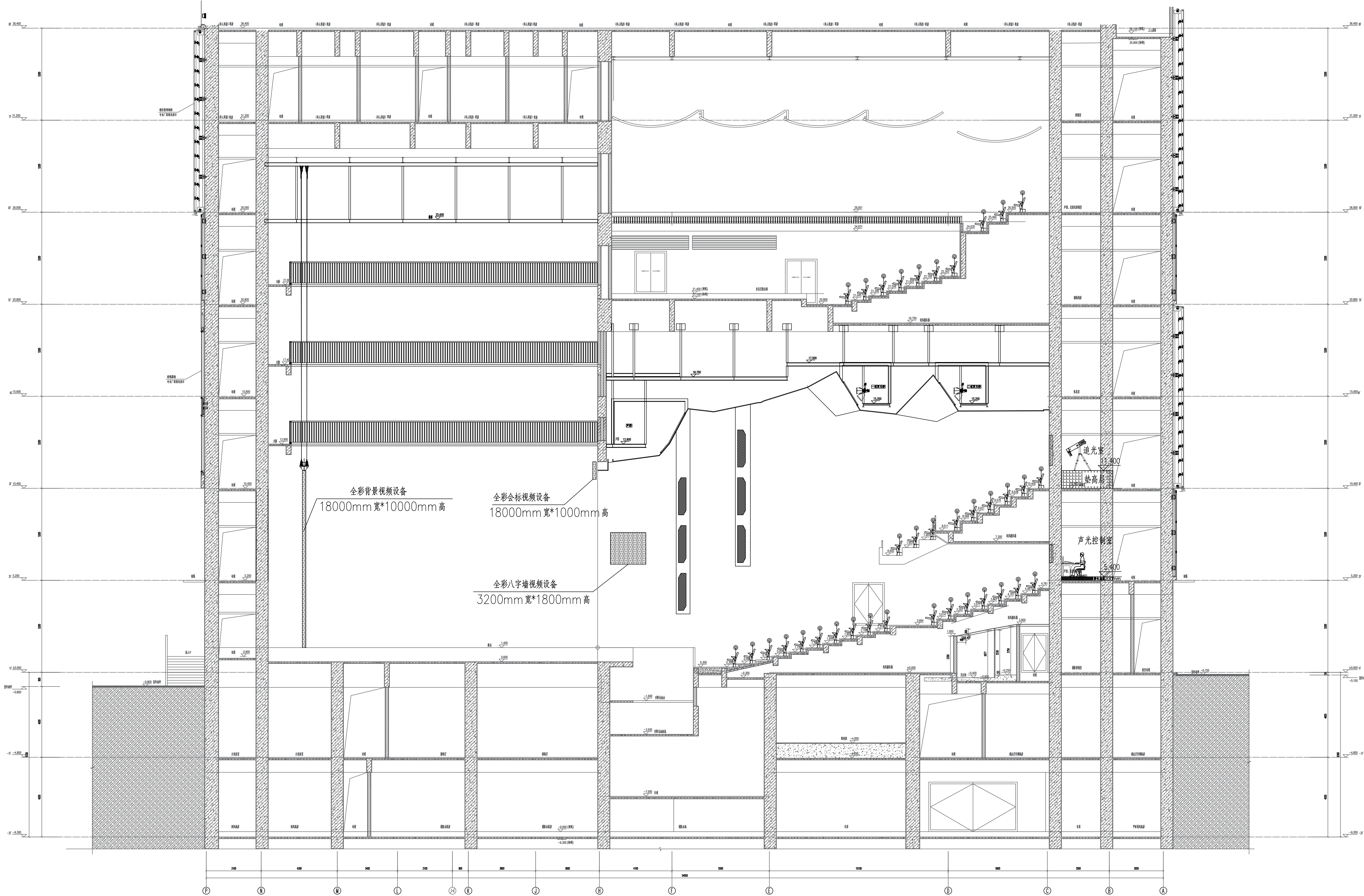
1-1剖面图
