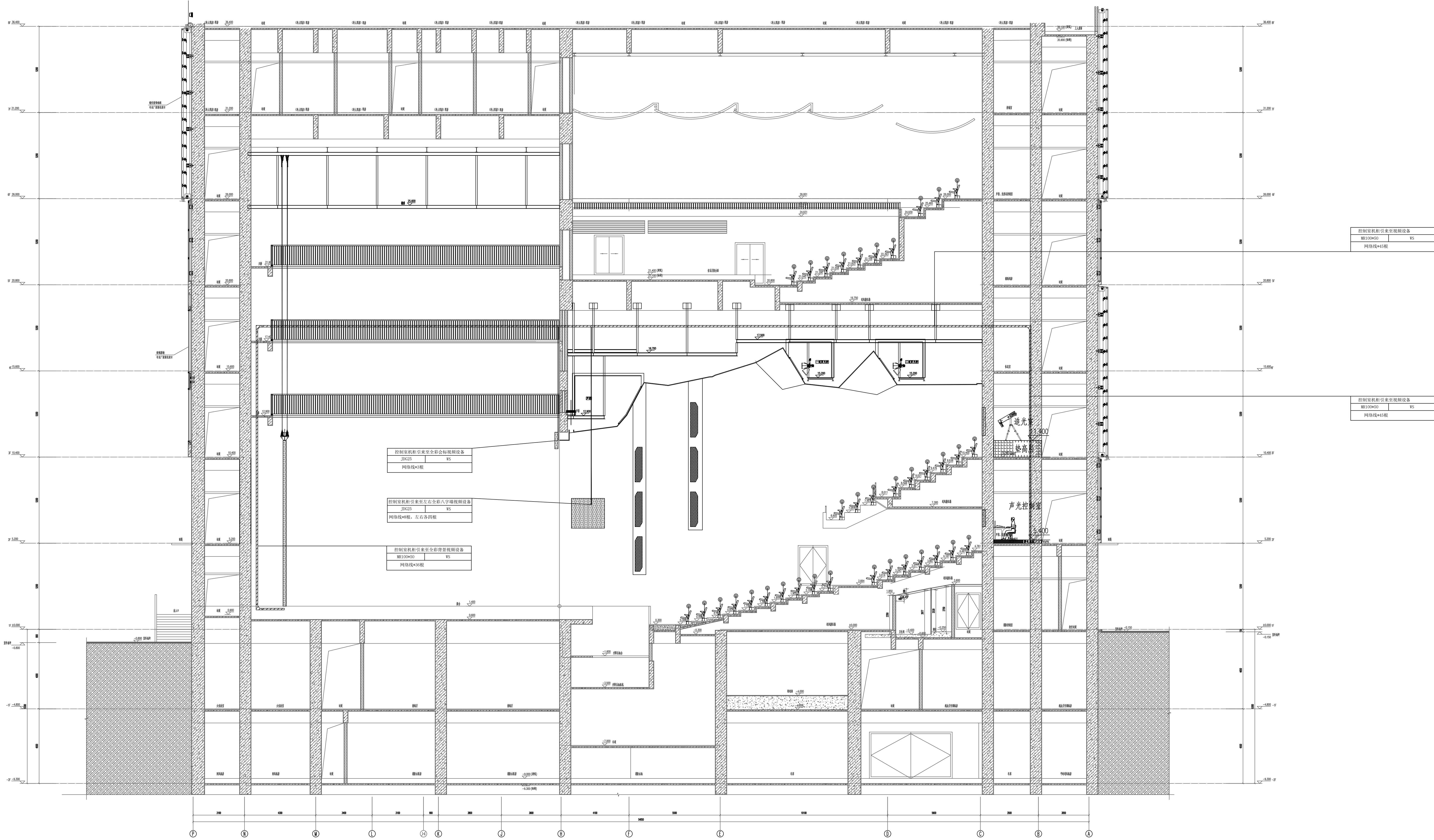
1-1剖面图
