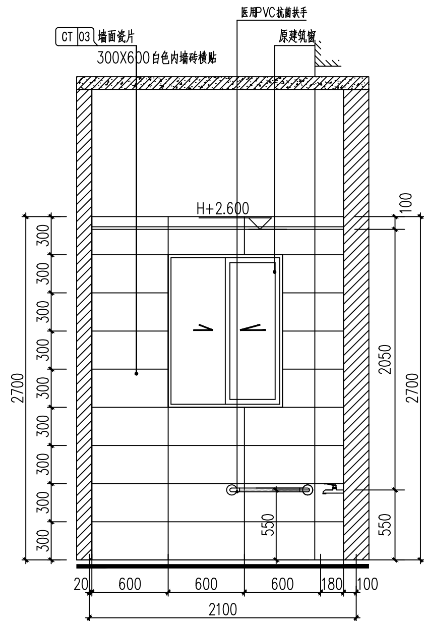
四、七层三人间病房卫生间C立面图 1:30
