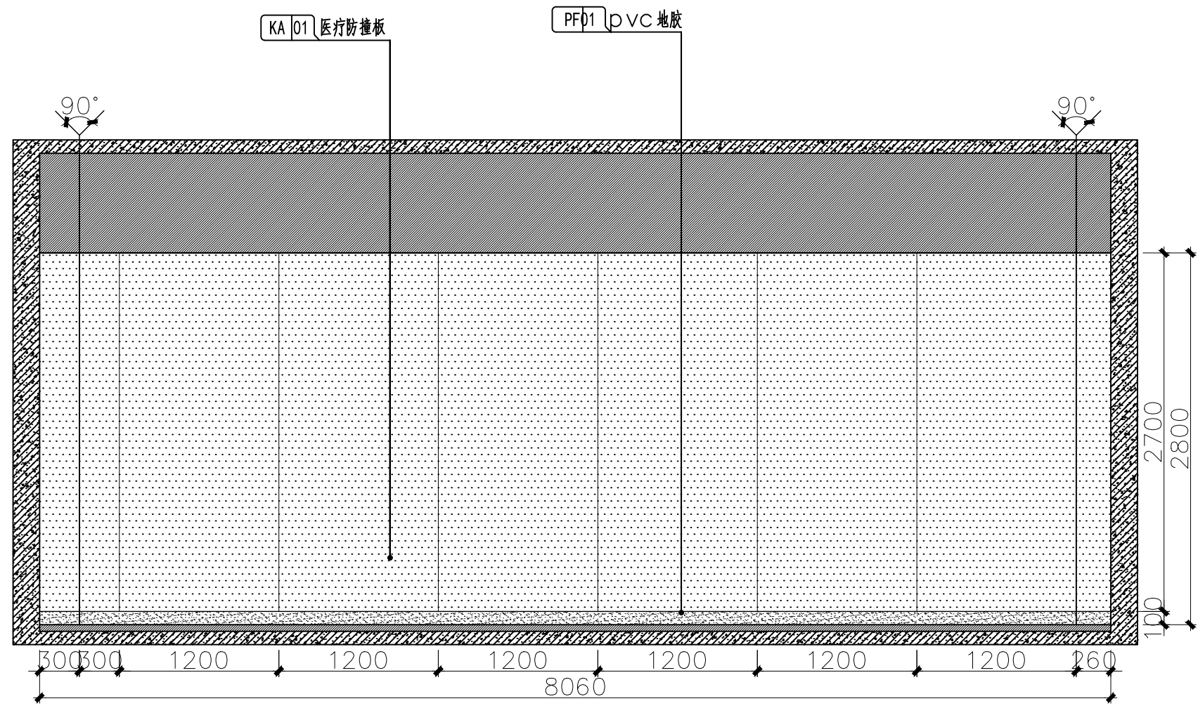
二层推拿治疗室B立面图 1:40
