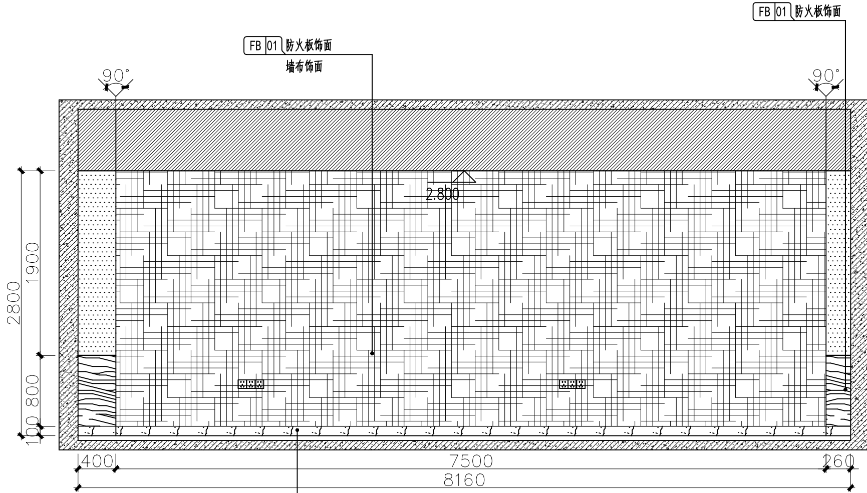
三层运动治疗大厅B立面图 1:40
