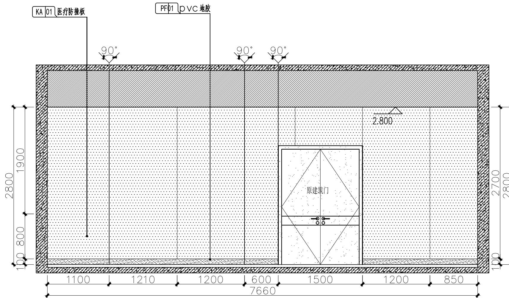
二层康复治疗师办公室A立面图 1:40
