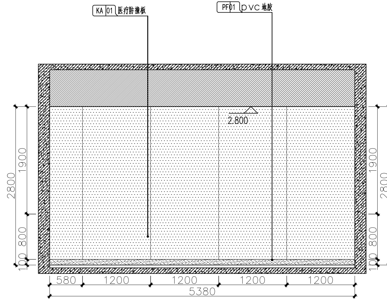
二层康复治疗师办公室B立面图 1:40
