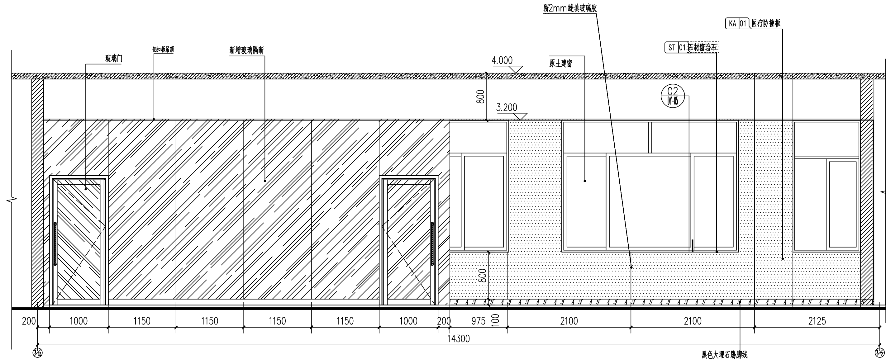
一层输液大厅C立面图 1:40
