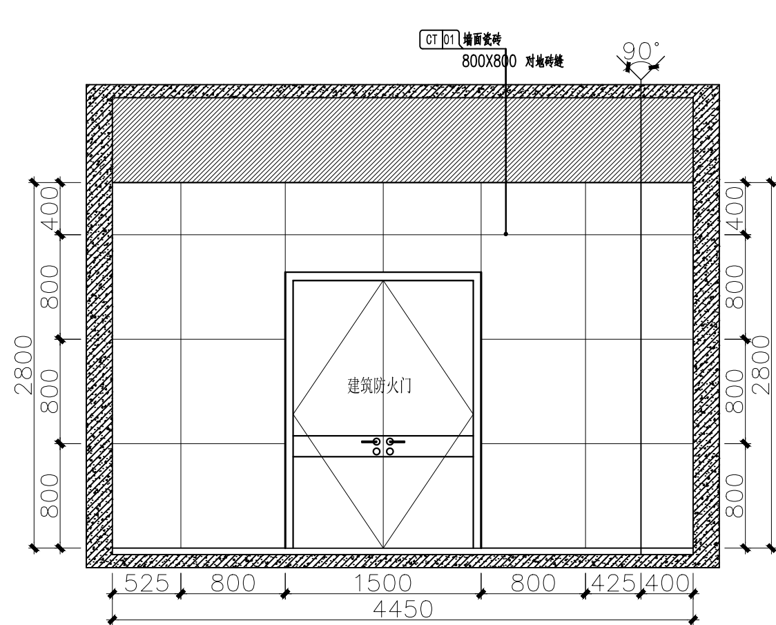
二层候梯厅C立面图 1:40
