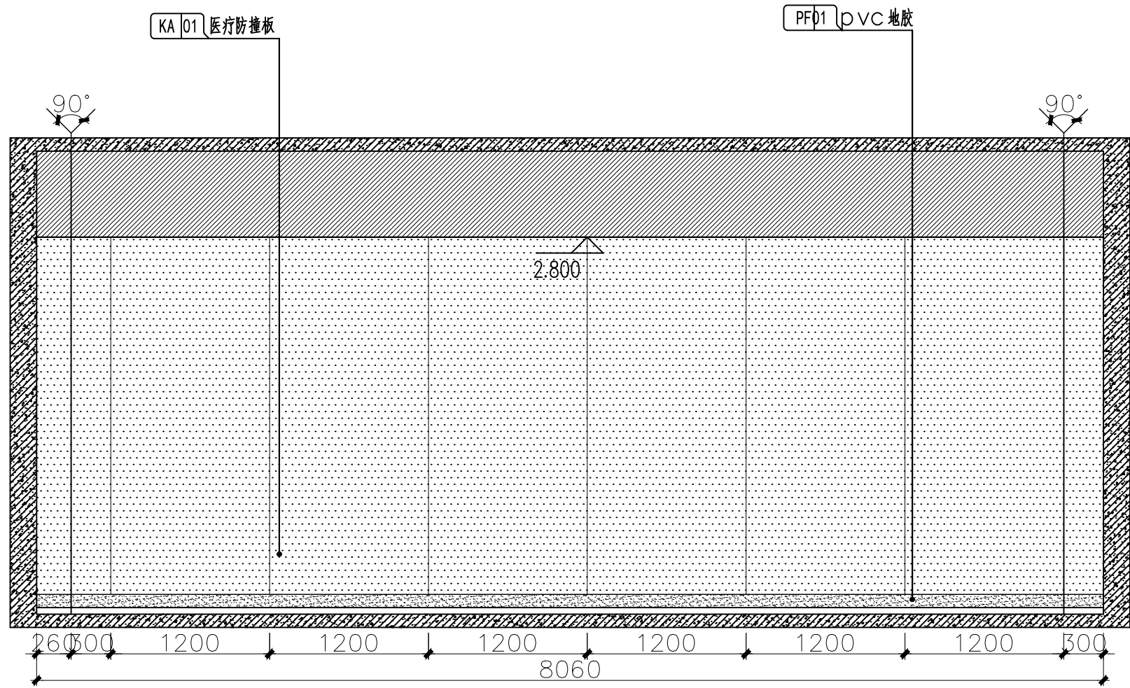
三层治疗室B立面图 1:40
