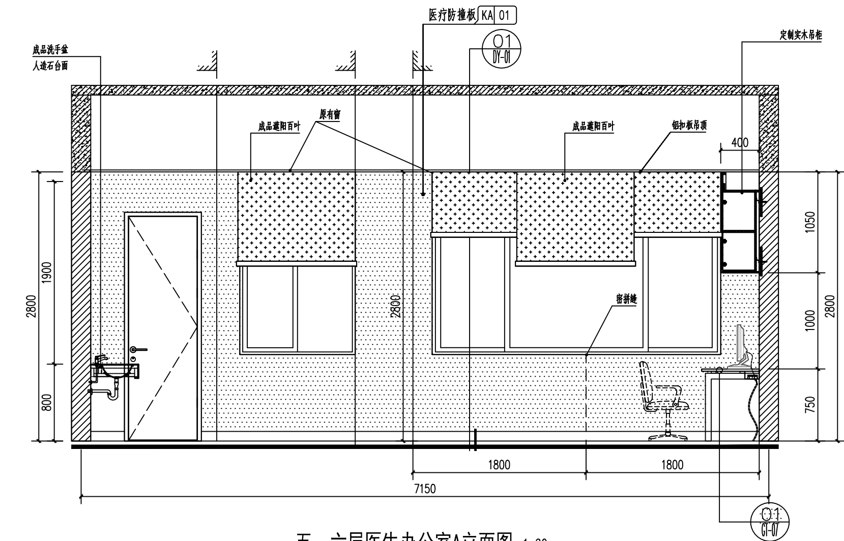
五、六层医生办公室A立面图 1:30
