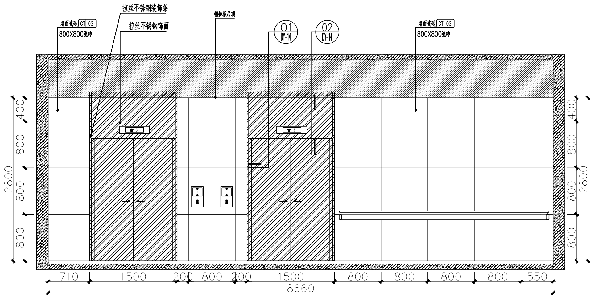
二层候梯厅B立面图 1:40
