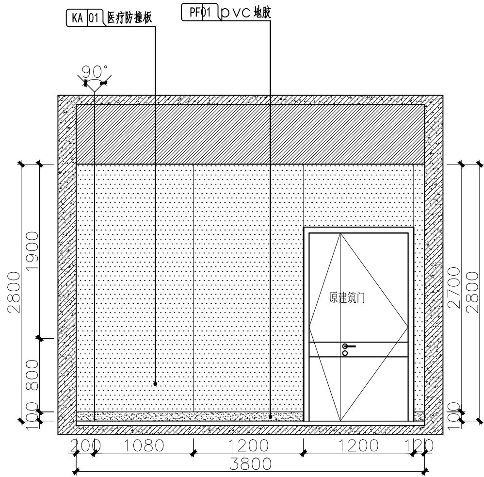
三层治疗室A立面图 1:40
