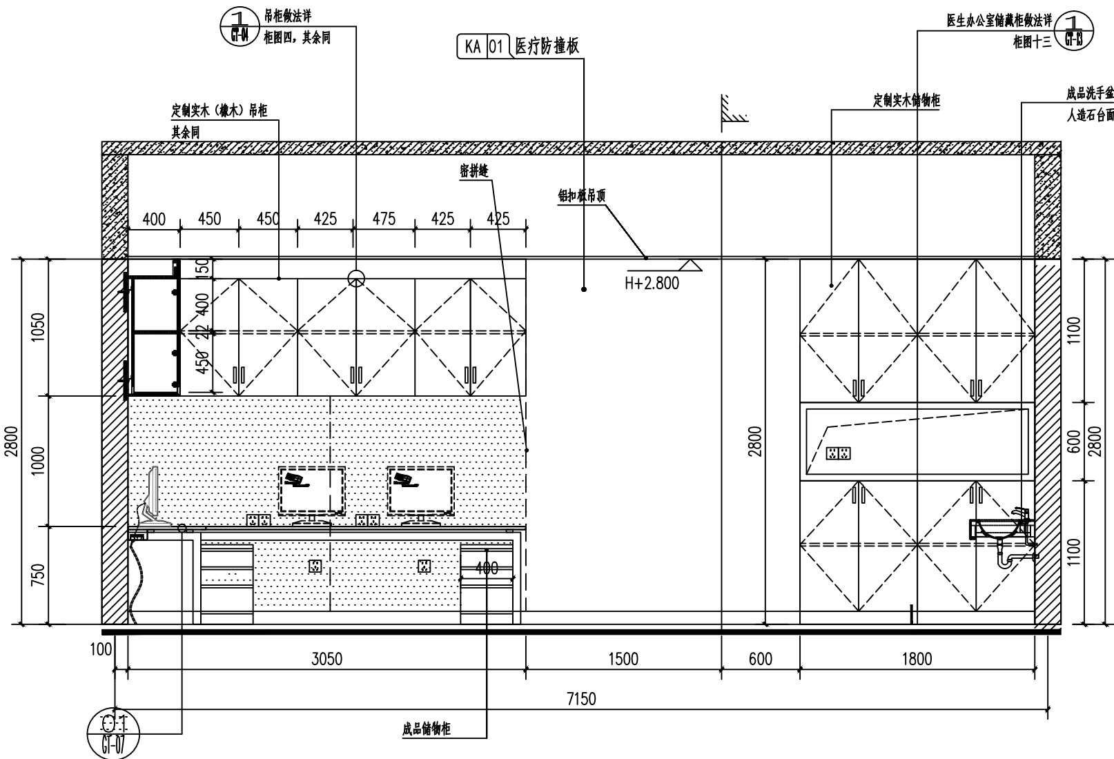
五、六层医生办公室C立面图 1:30
