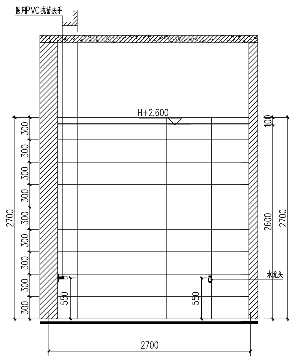
四、七层三人间病房卫生间B立面图 1:30
