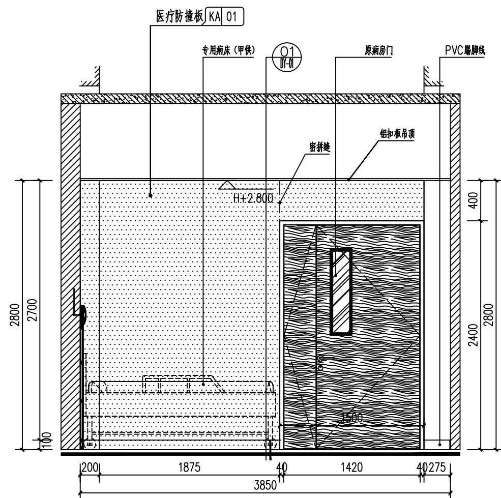
四、七层三人间病房A立面图 1:30
