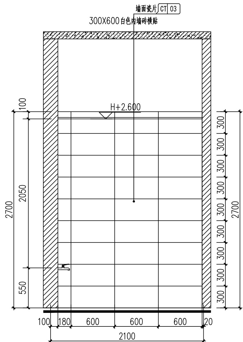
四、七层三人间病房卫生间A立面图 1:30
