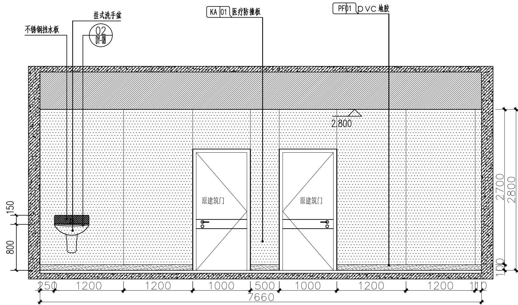
二层康复治疗师办公室C立面图 1:40
