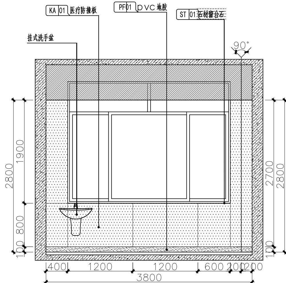
三层治疗室C立面图 1:40
