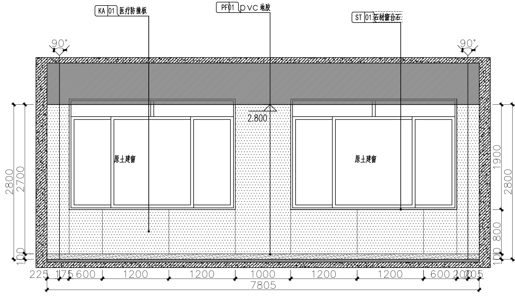
二层推拿治疗室C立面图 1:40
