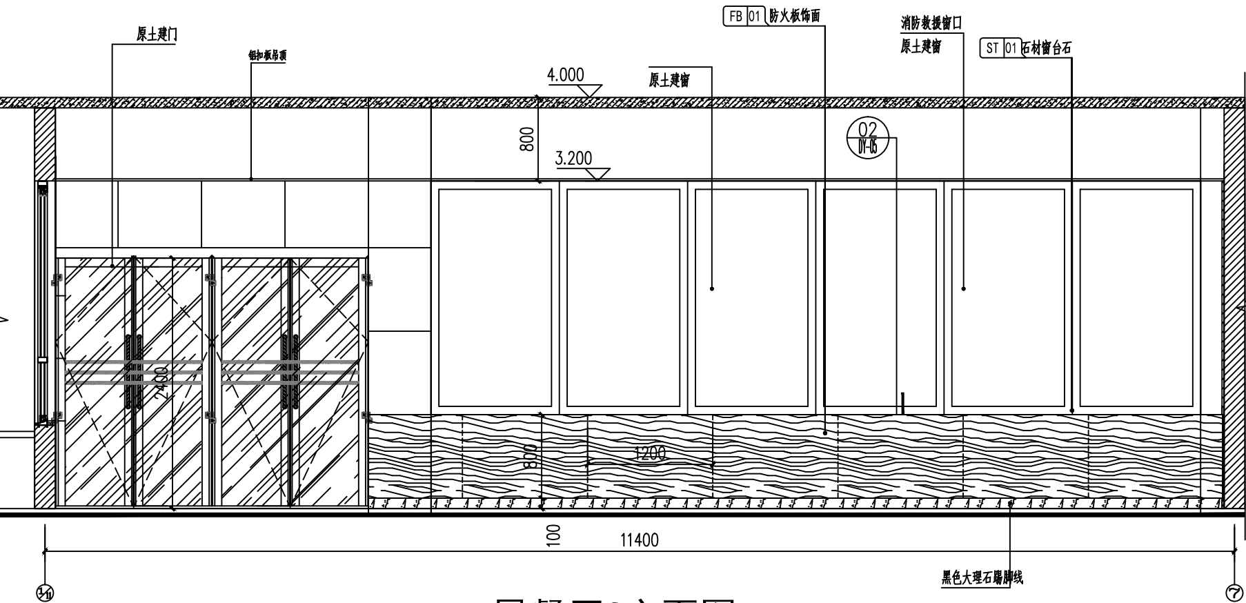
一层餐厅C立面图 1:40
