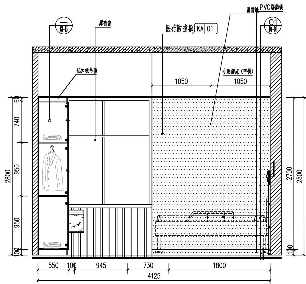
三层三人间病房C立面图 1:30
