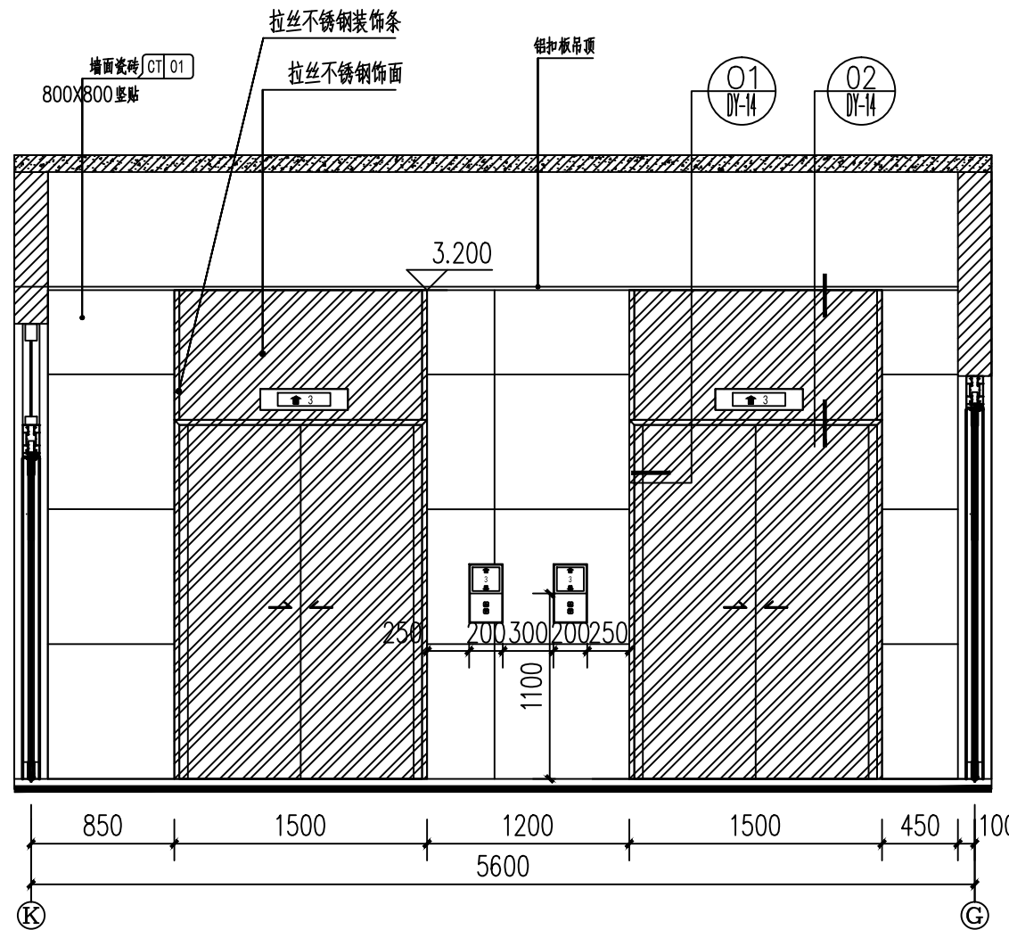
一层候梯厅D立面图 1:40
