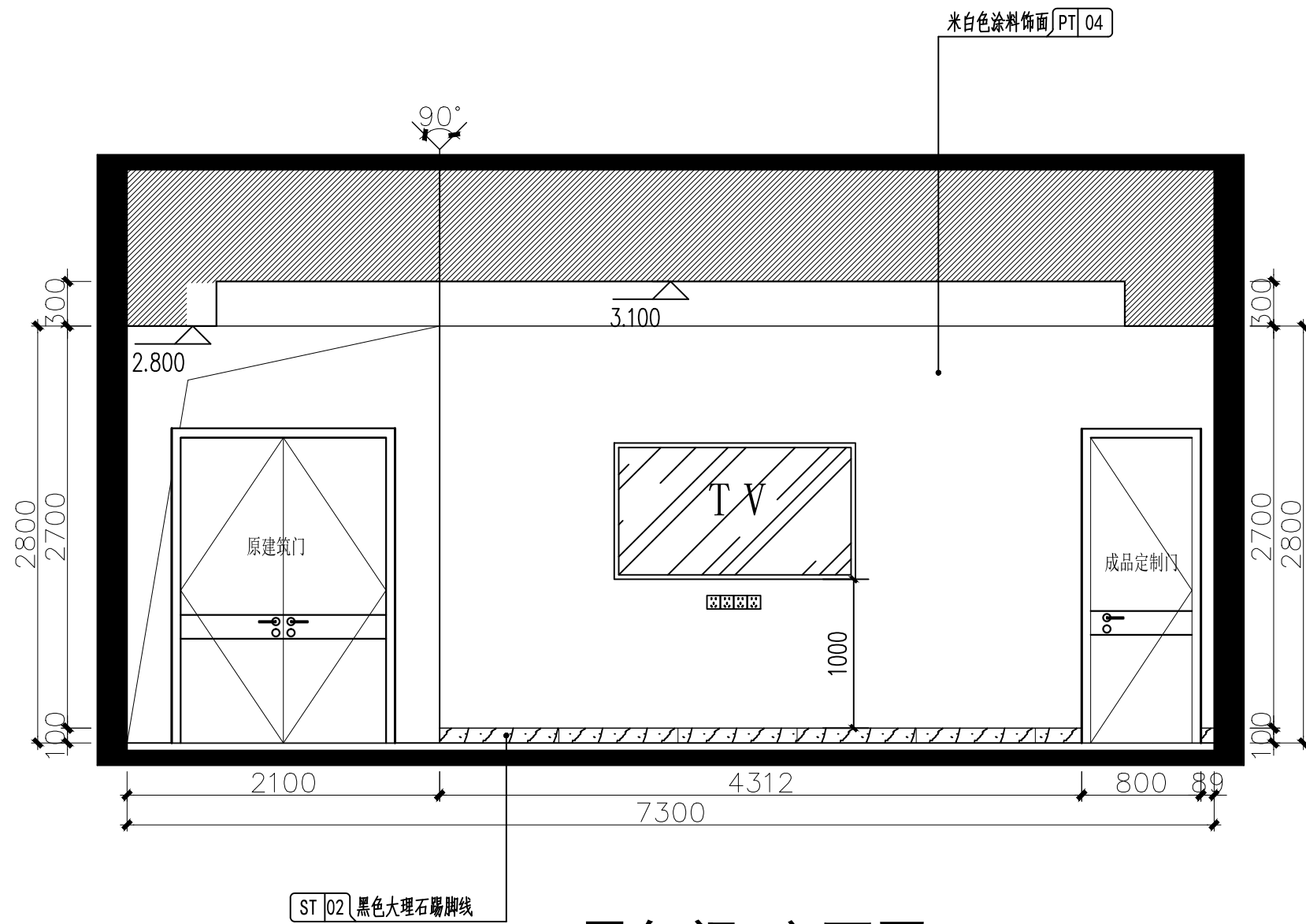
一层包间C立面图 1:40
