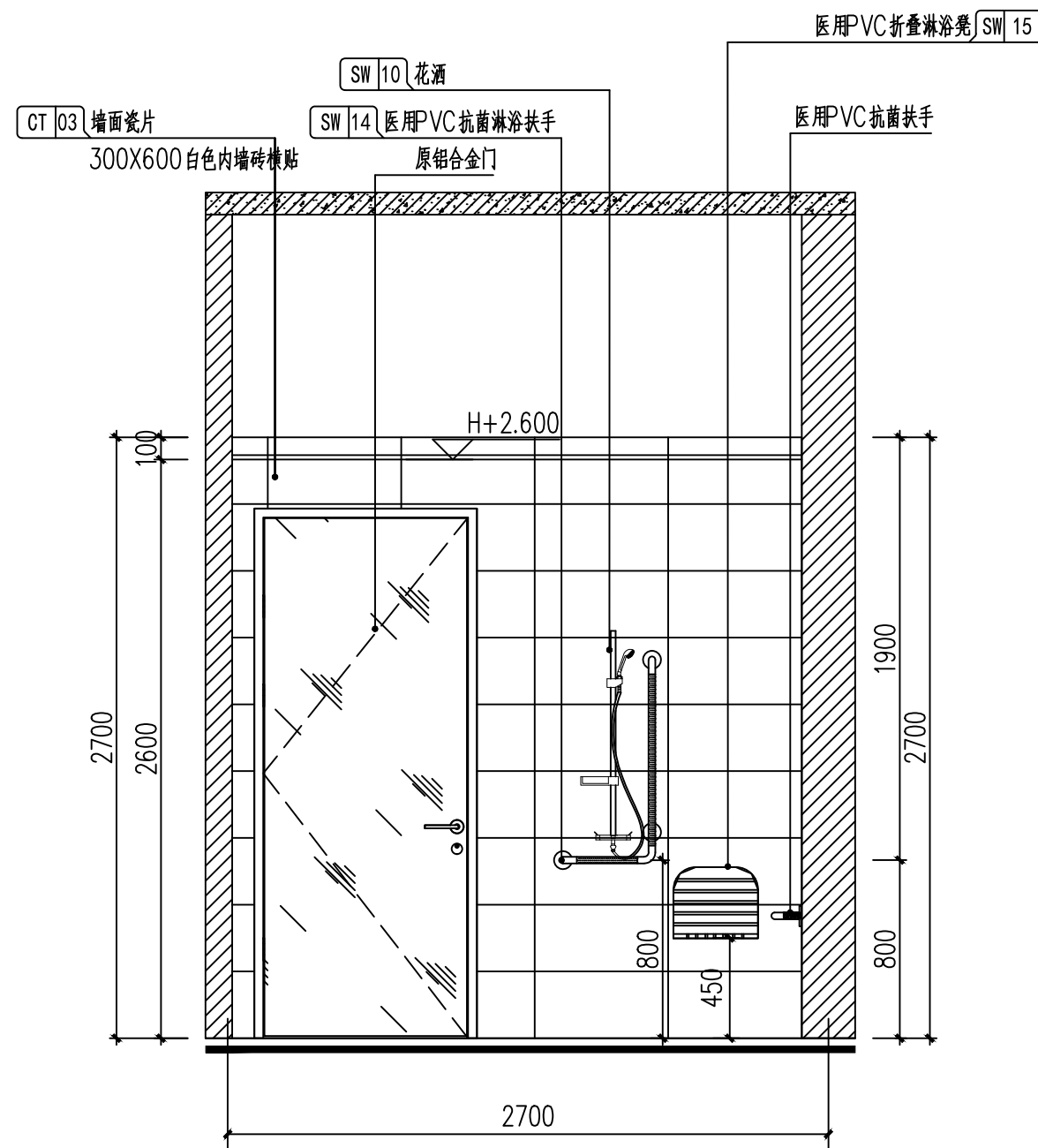
四、七层三人间病房卫生间D立面图 1:30
