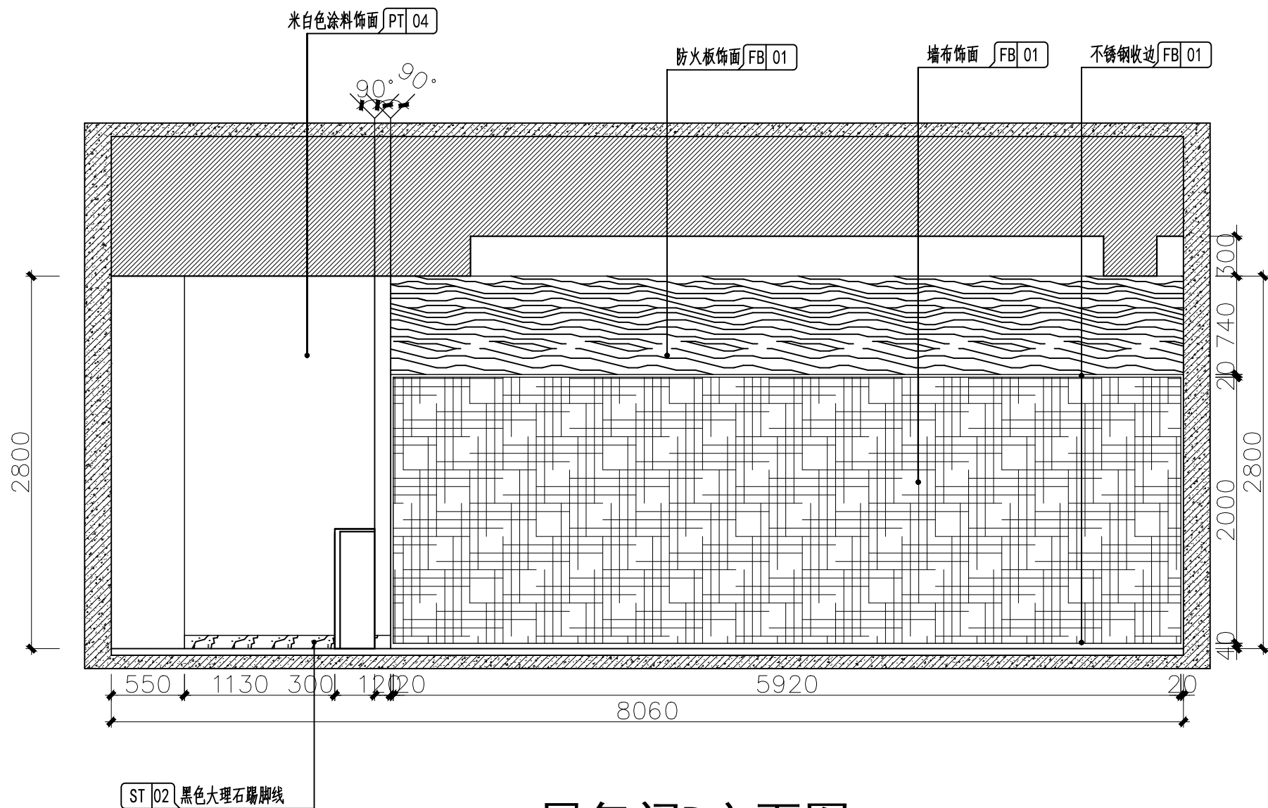
一层包间D立面图 1:40
