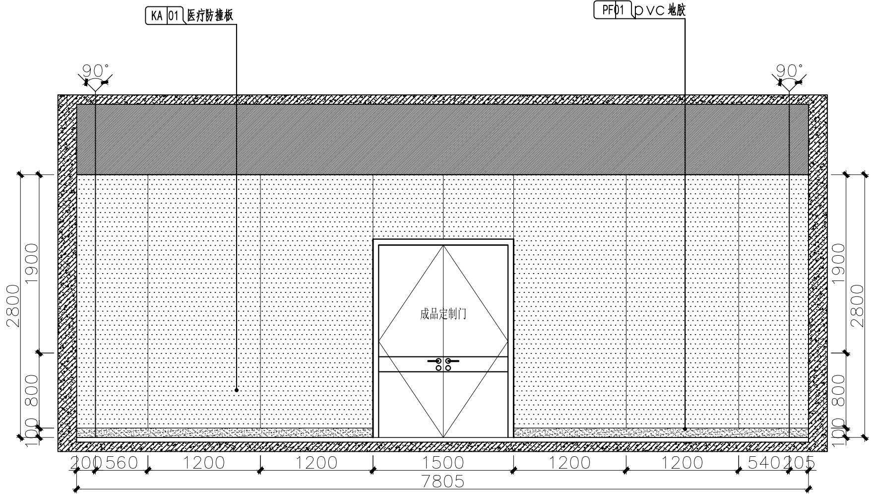
二层推拿治疗室A立面图 1:40
