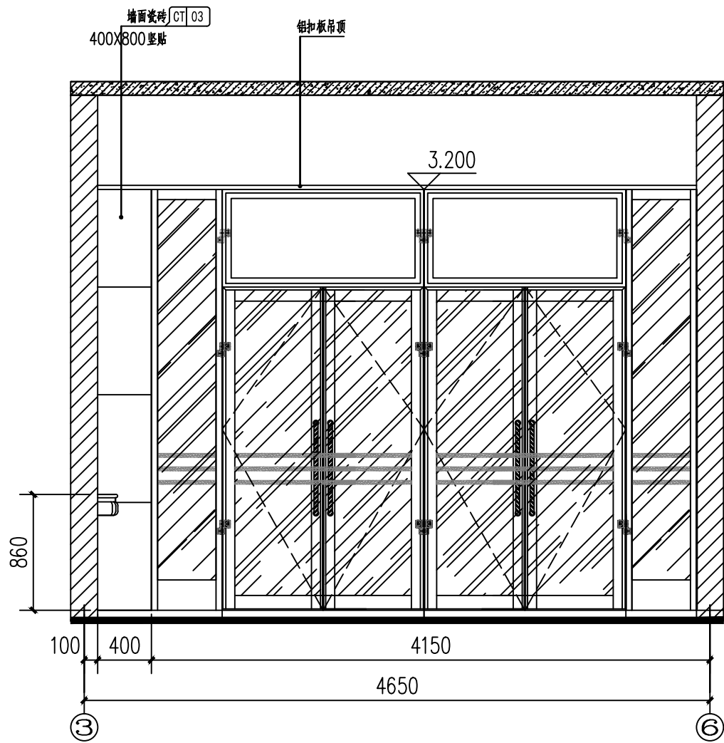
一层候梯厅A立面图 1:40
