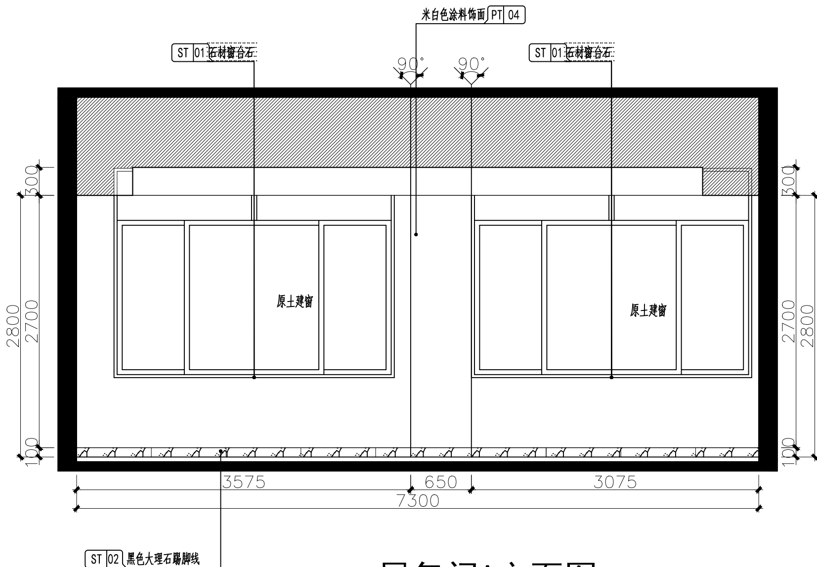
一层包间A立面图 1:40
