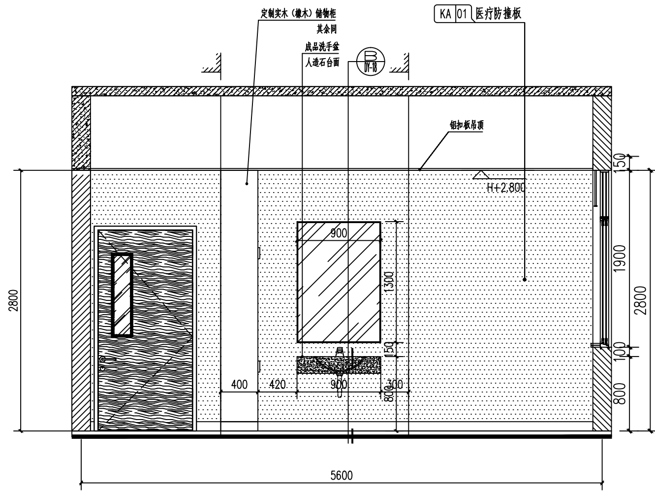
五、六层医生办公室B立面图 1:30
