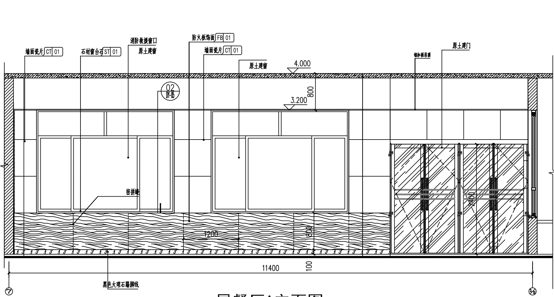
一层餐厅A立面图 1:40
