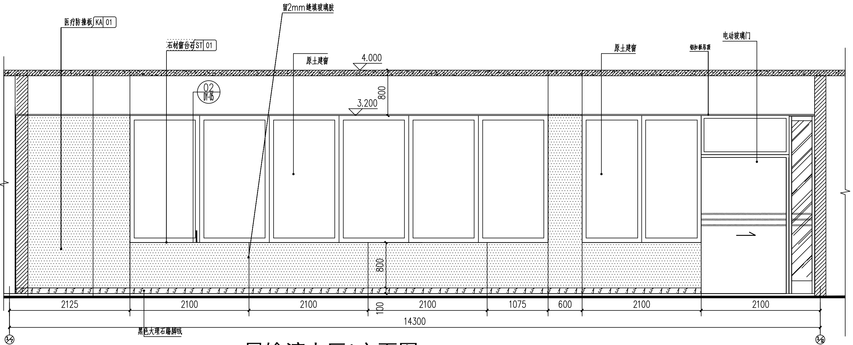
一层输液大厅A立面图 1:40
