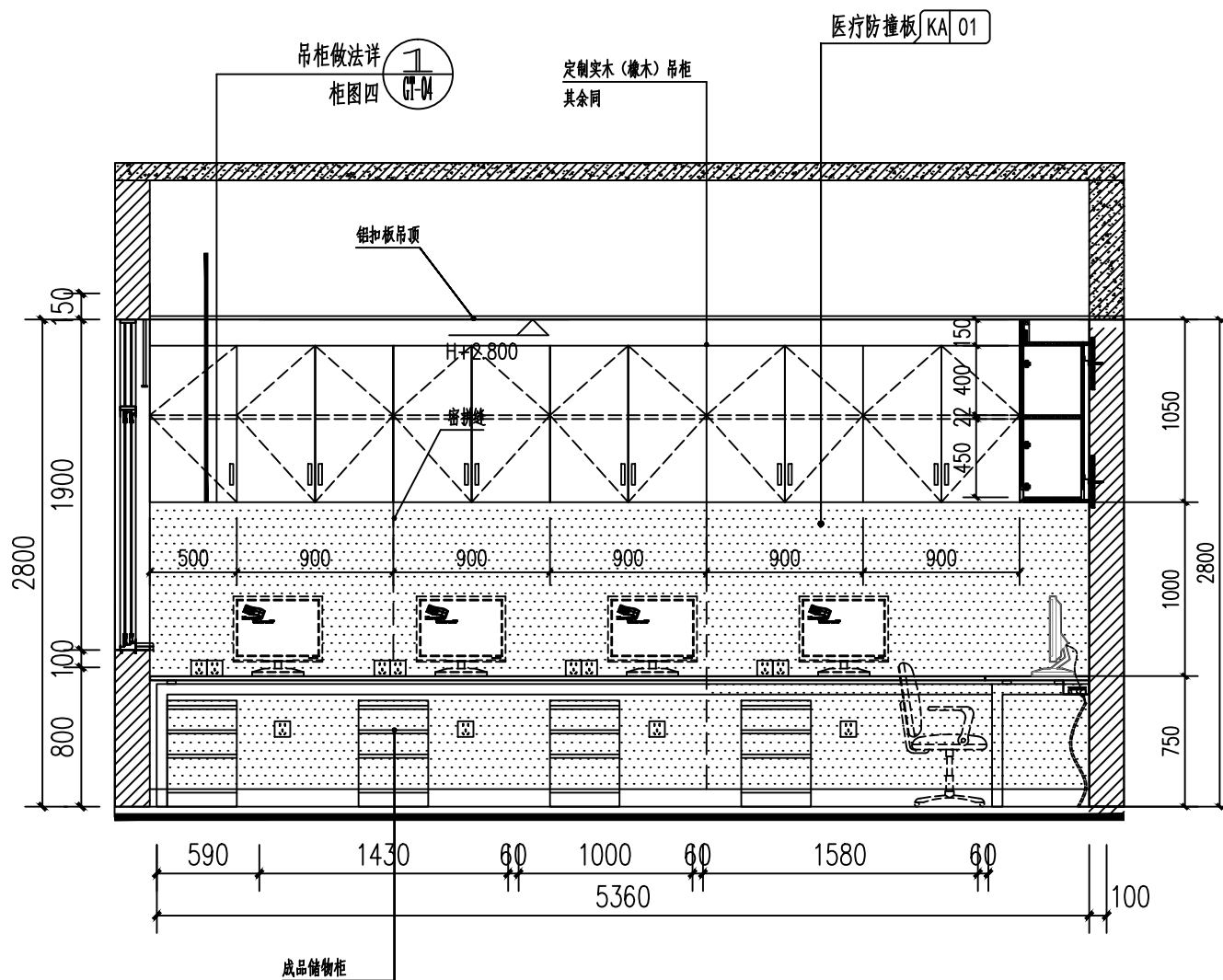
五、六层医生办公室D立面图 1:30
