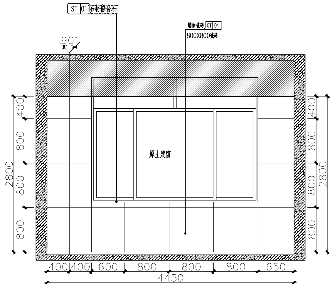
二层候梯厅A立面图 1:40
