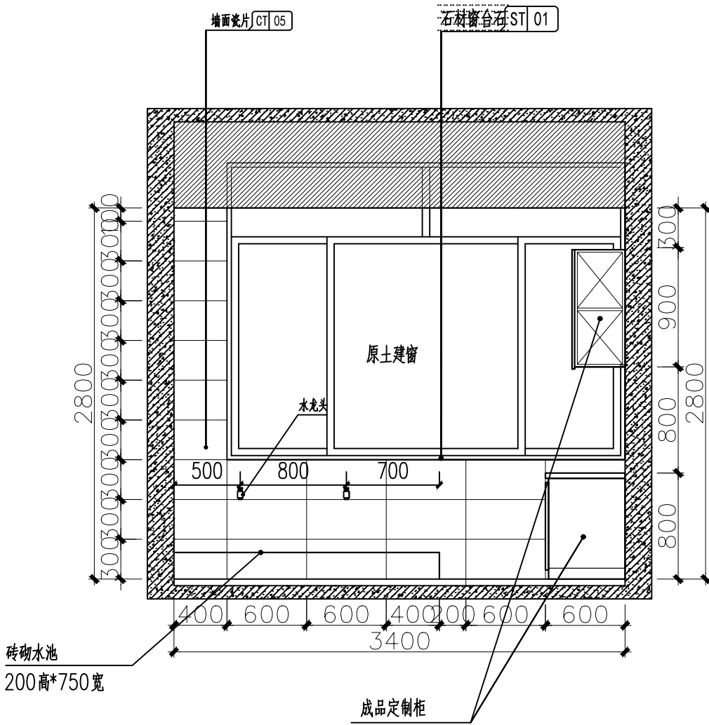
二层操作间B立面图 1:40
