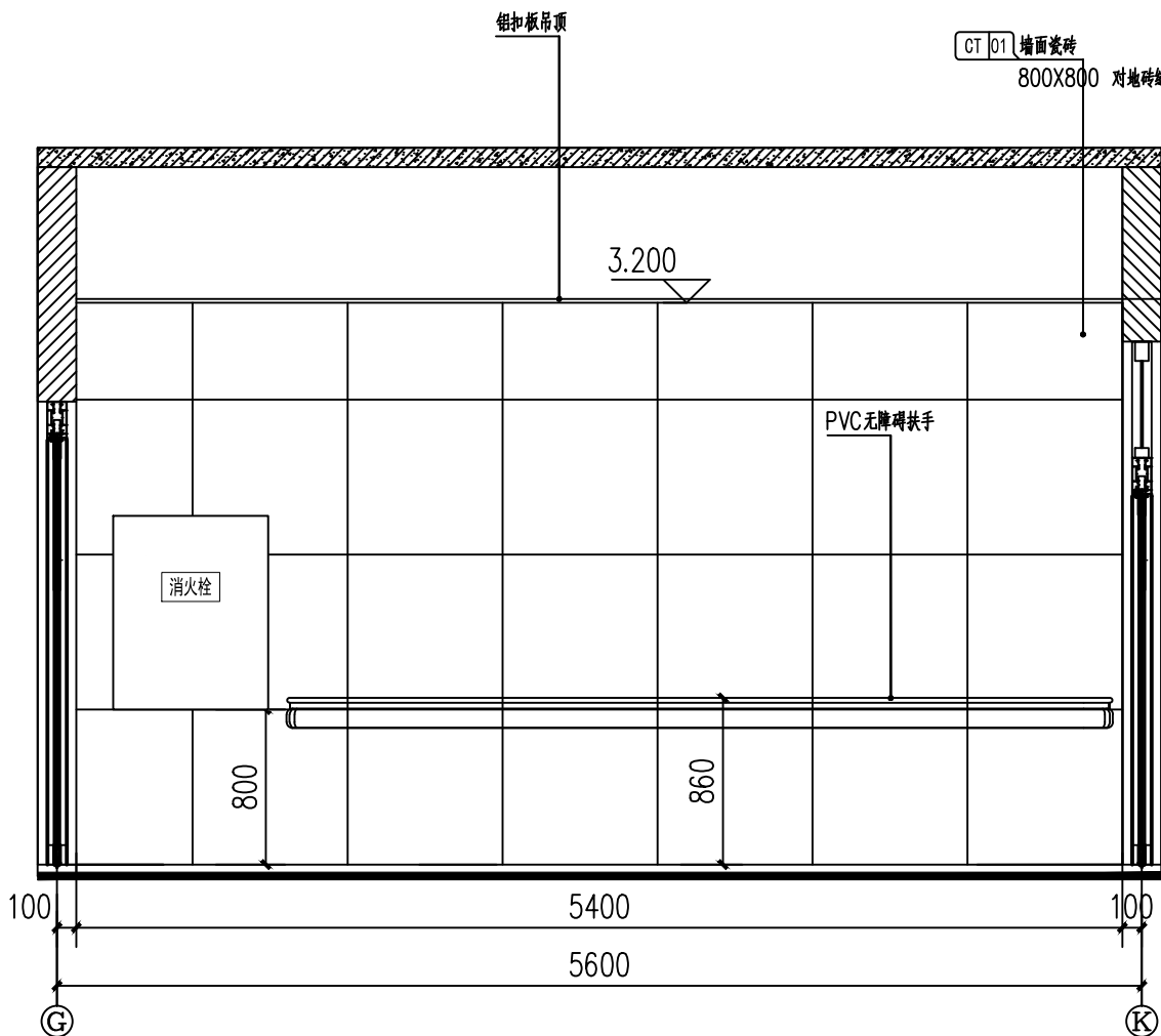
一层候梯厅B立面图 1:40
