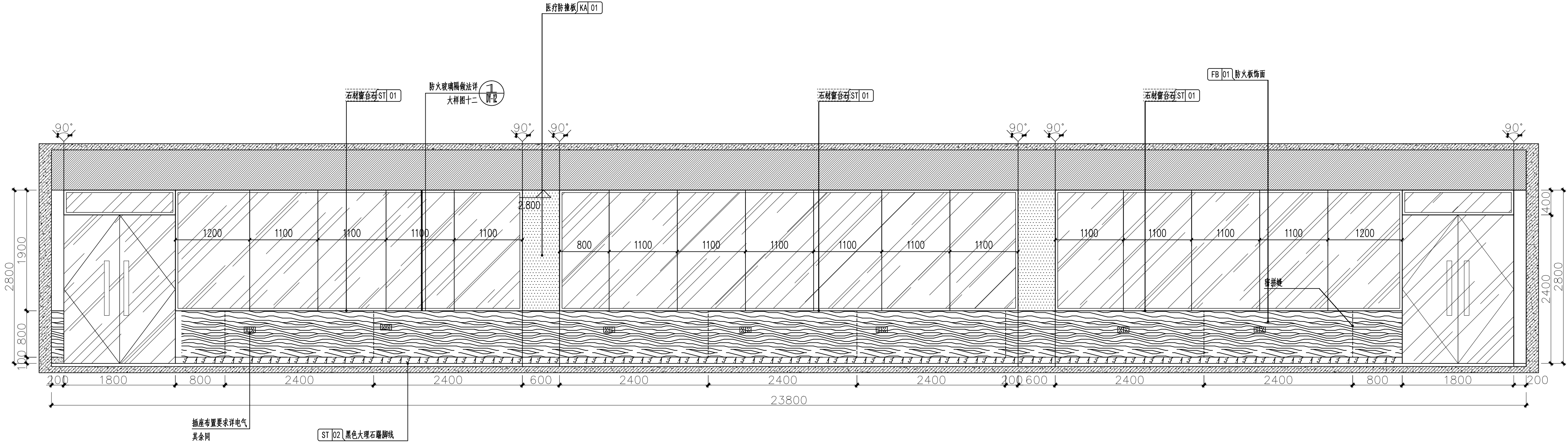
三层运动治疗大厅A立面图 1:40
