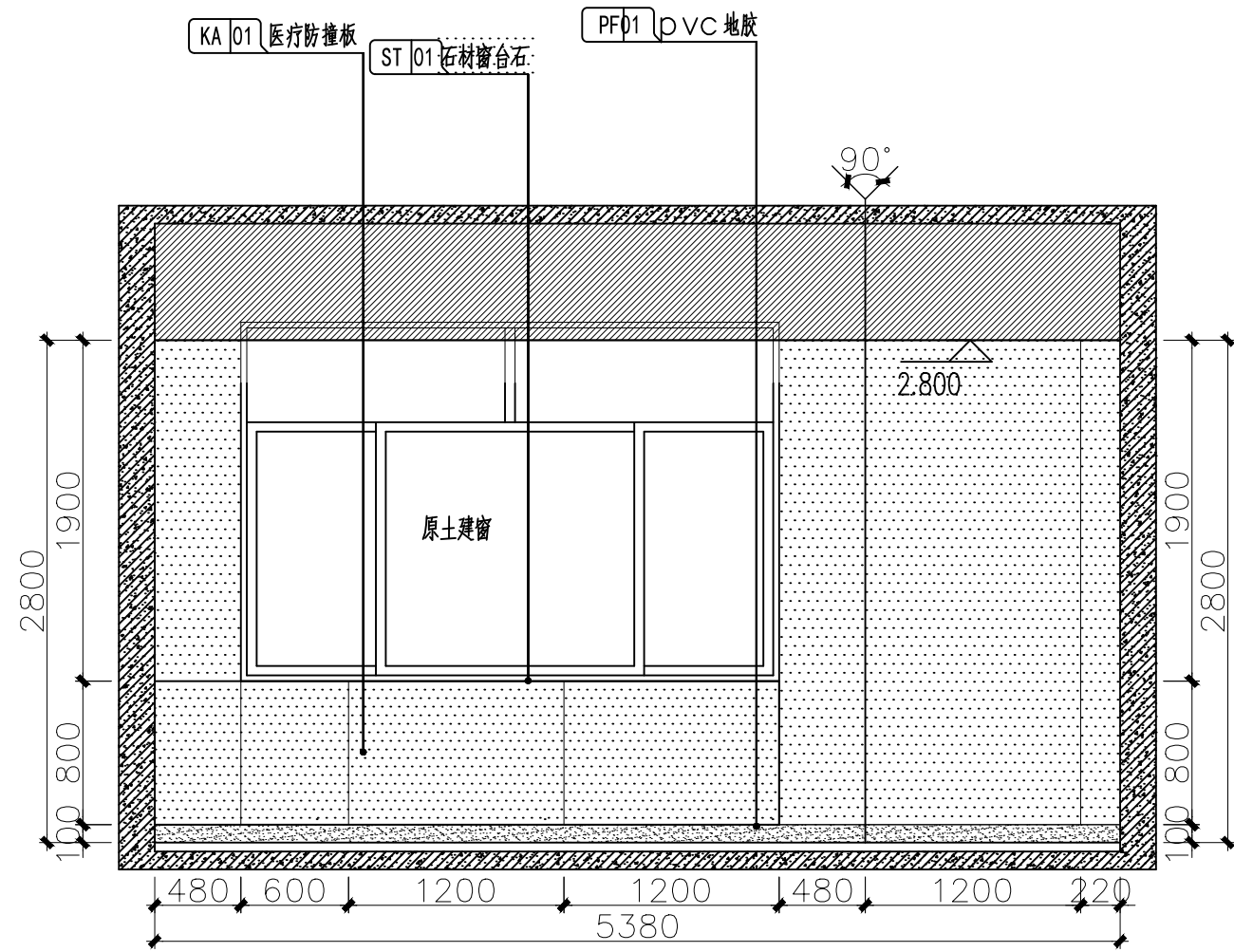
二层康复治疗师办公室D立面图 1:40
