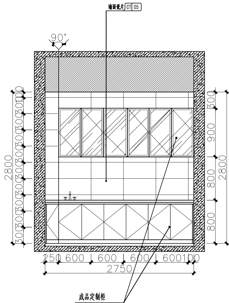
二层操作间A立面图 1:40
