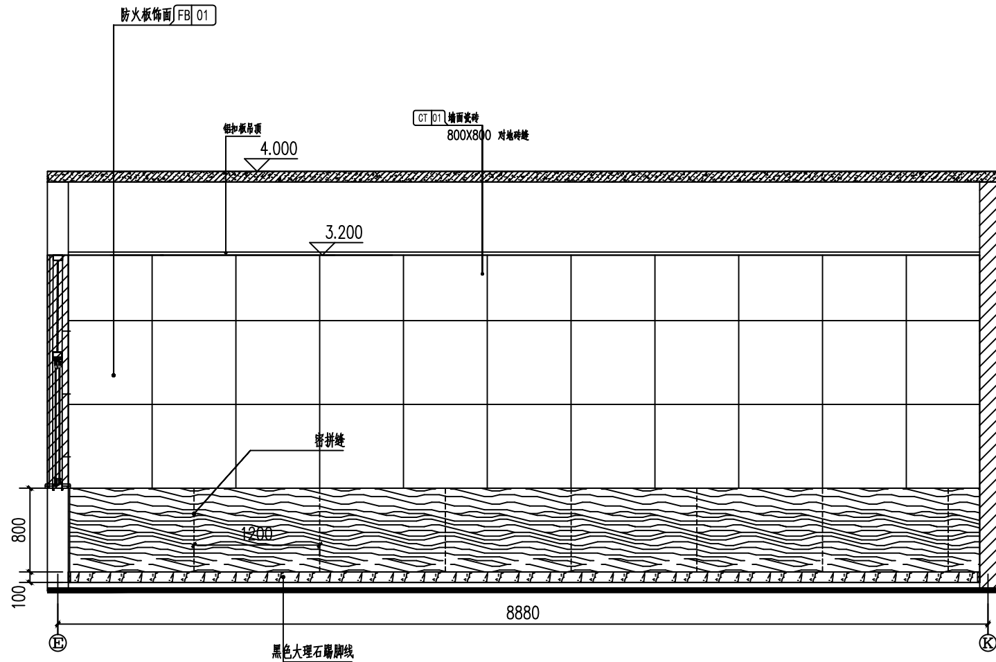
一层餐厅B立面图 1:40
