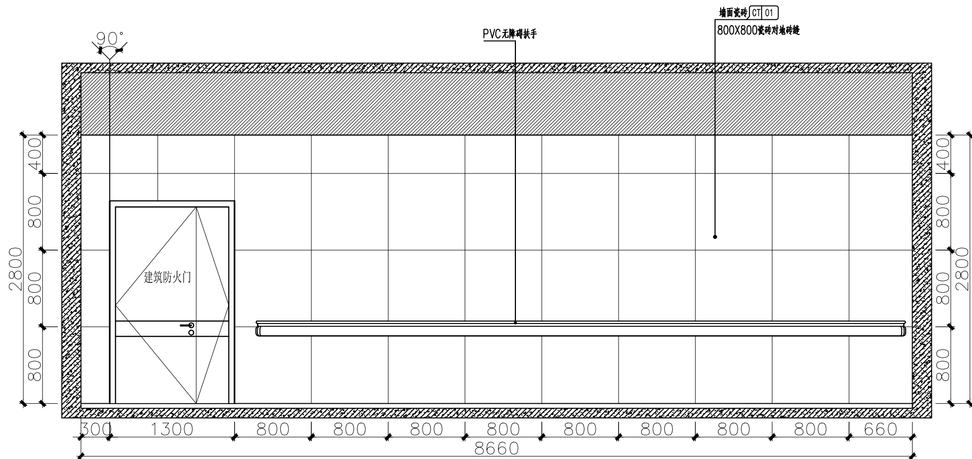
二层候梯厅D立面图 1:40
