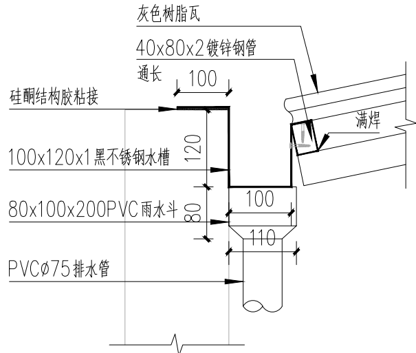
水槽做法大样 1:10
