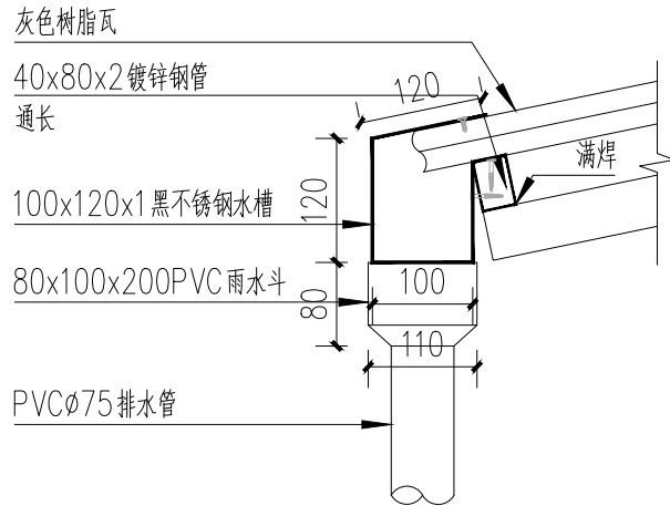
水槽做法大样 1:10
