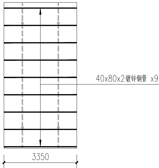
4号楼屋面檩条平面图 1:100
