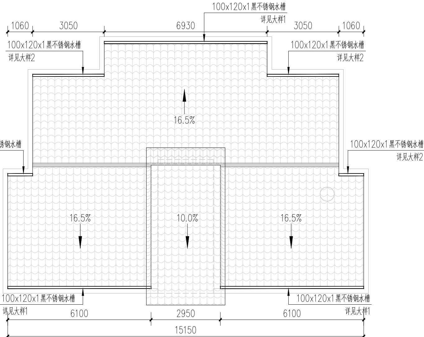
4号楼屋面屋顶平面图 1:100
