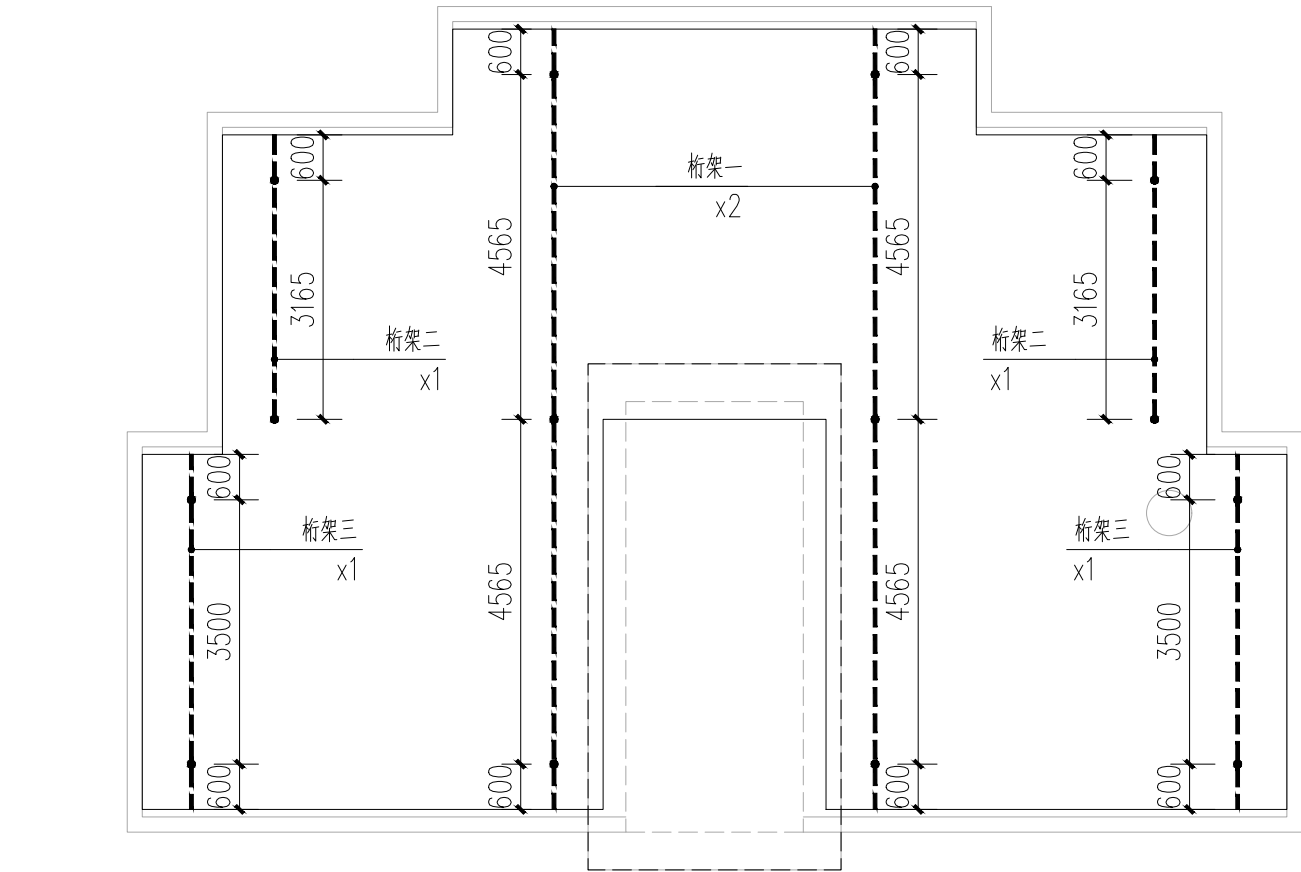
4号楼屋面立柱平面图 1:100
