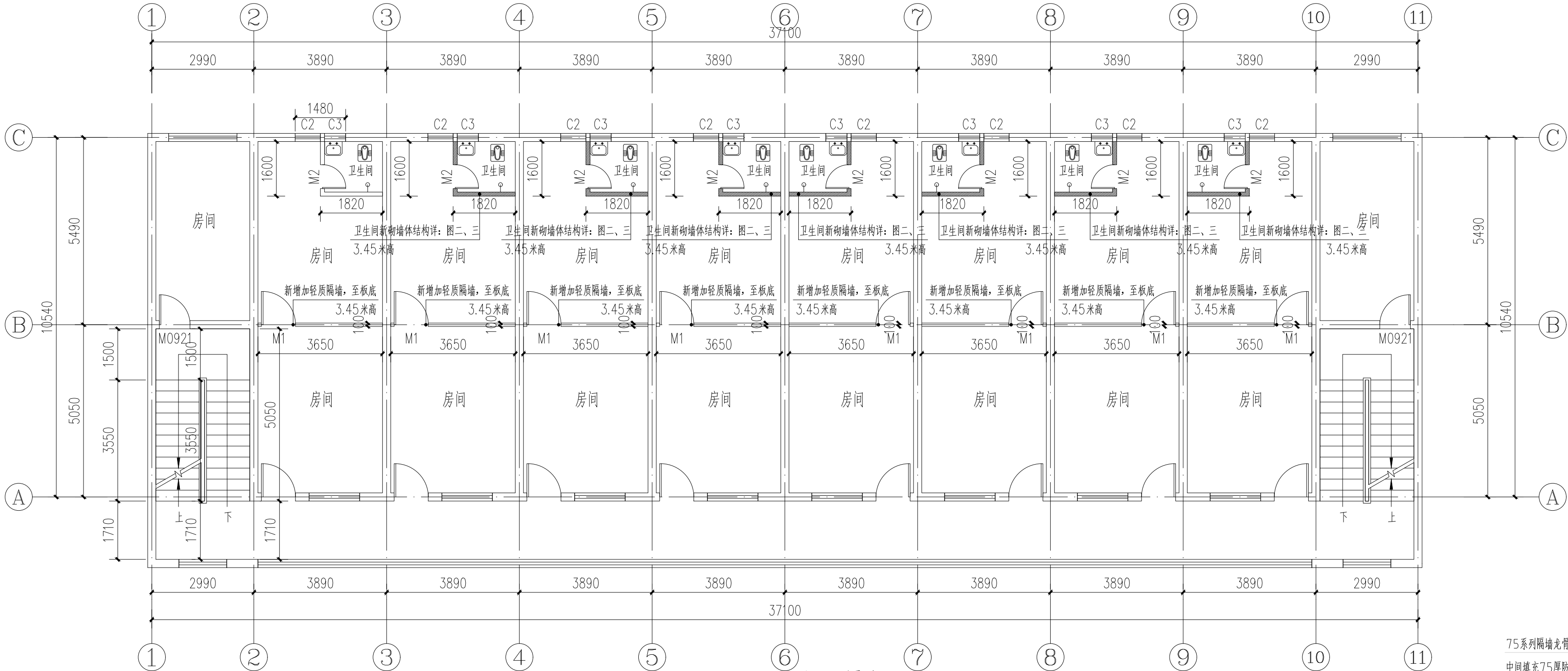
1号楼二层隔墙设计平面图 1:100
