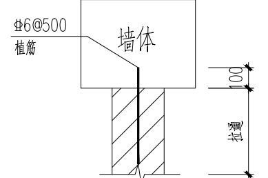
图二：墙拉筋详图
