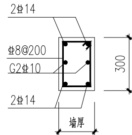
图三：圈梁详图 门楣圈梁
