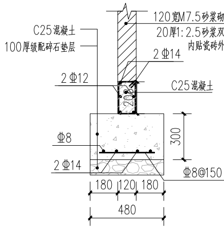
图一：一层卫生间隔墙基础图 1:20
