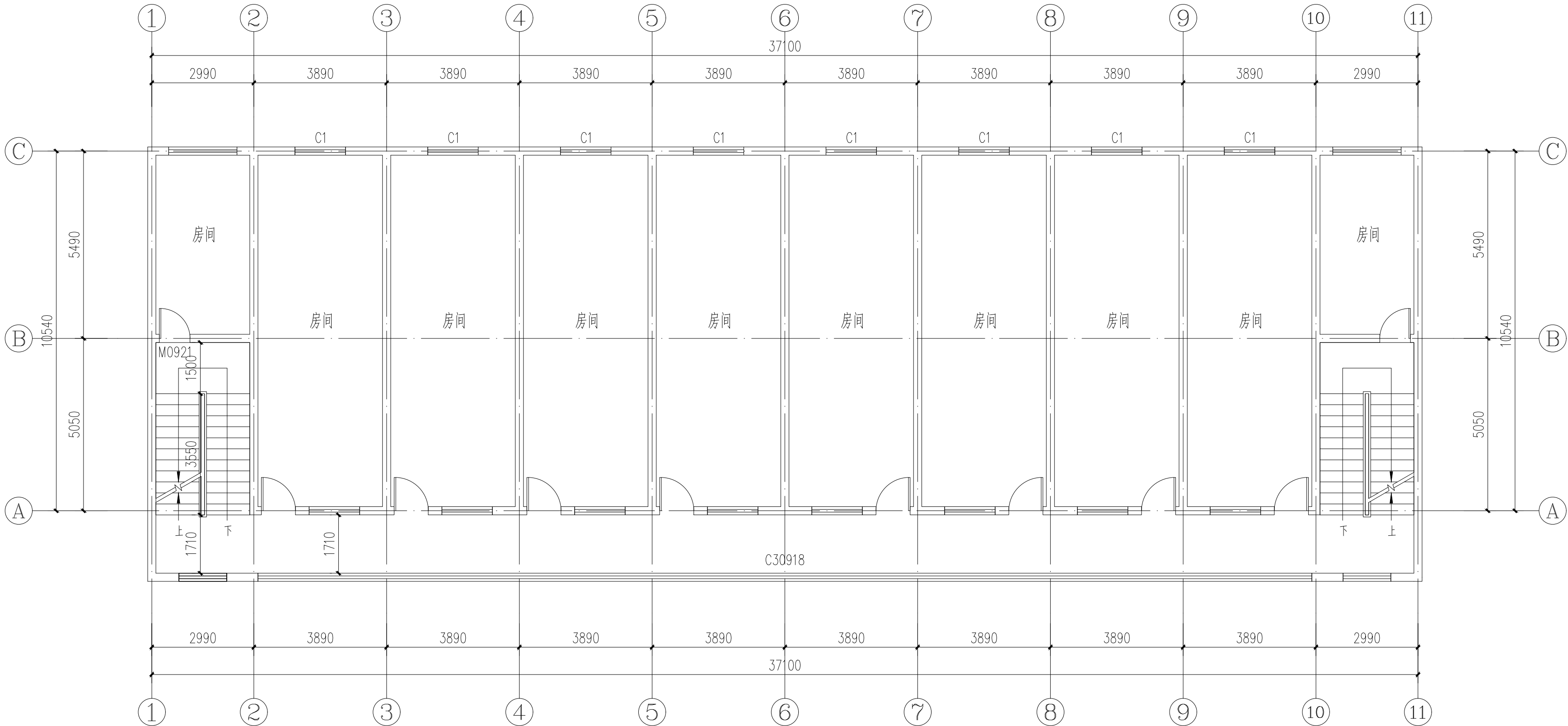
1号楼三层原始平面图 1:100
