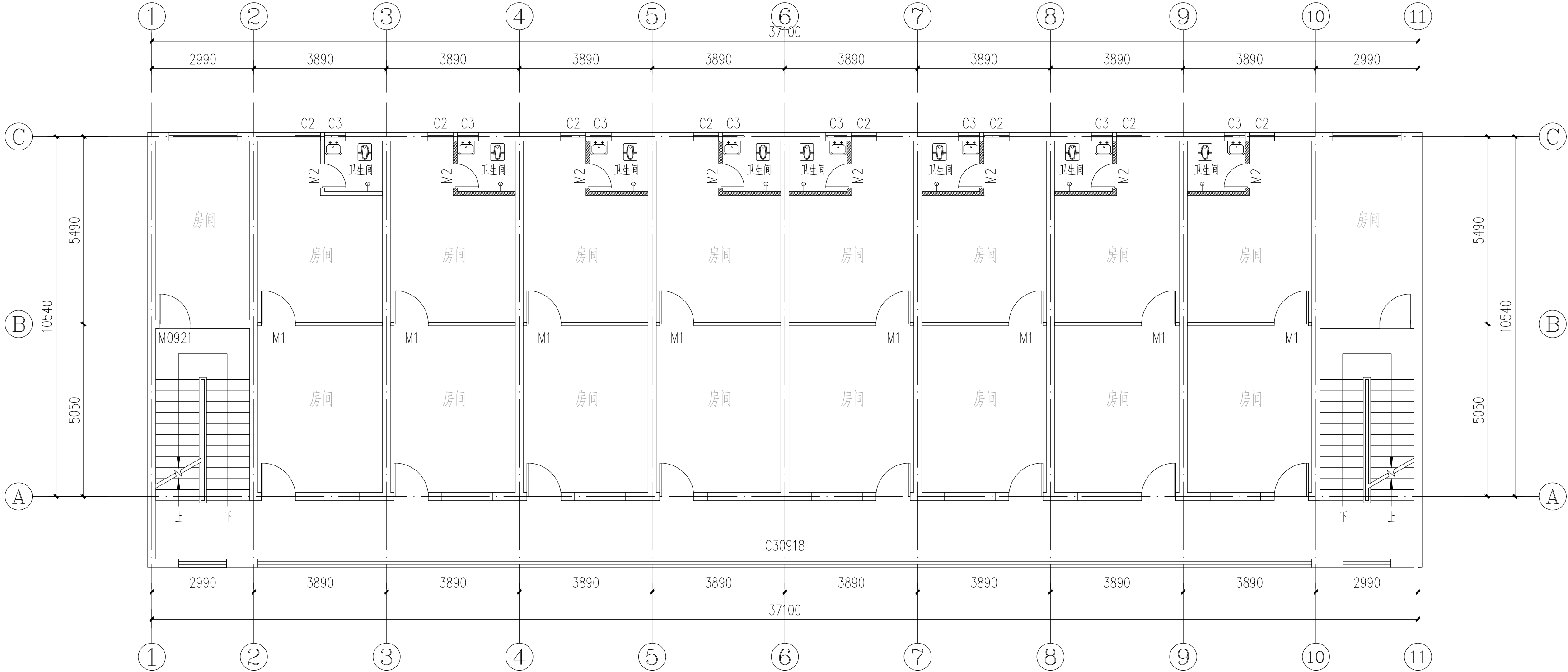
1号楼一层至三层门窗设计平面图 1:100
