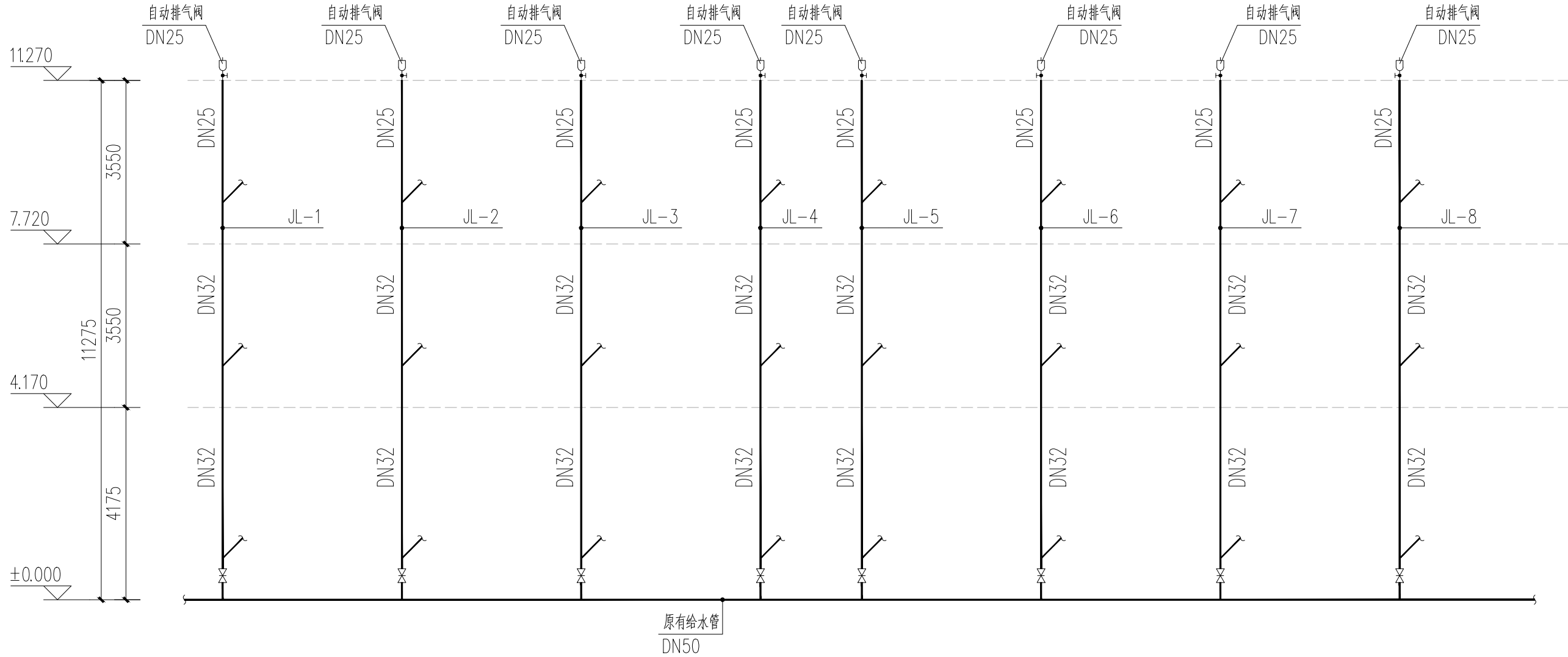
1号楼给水系统图 1:100
