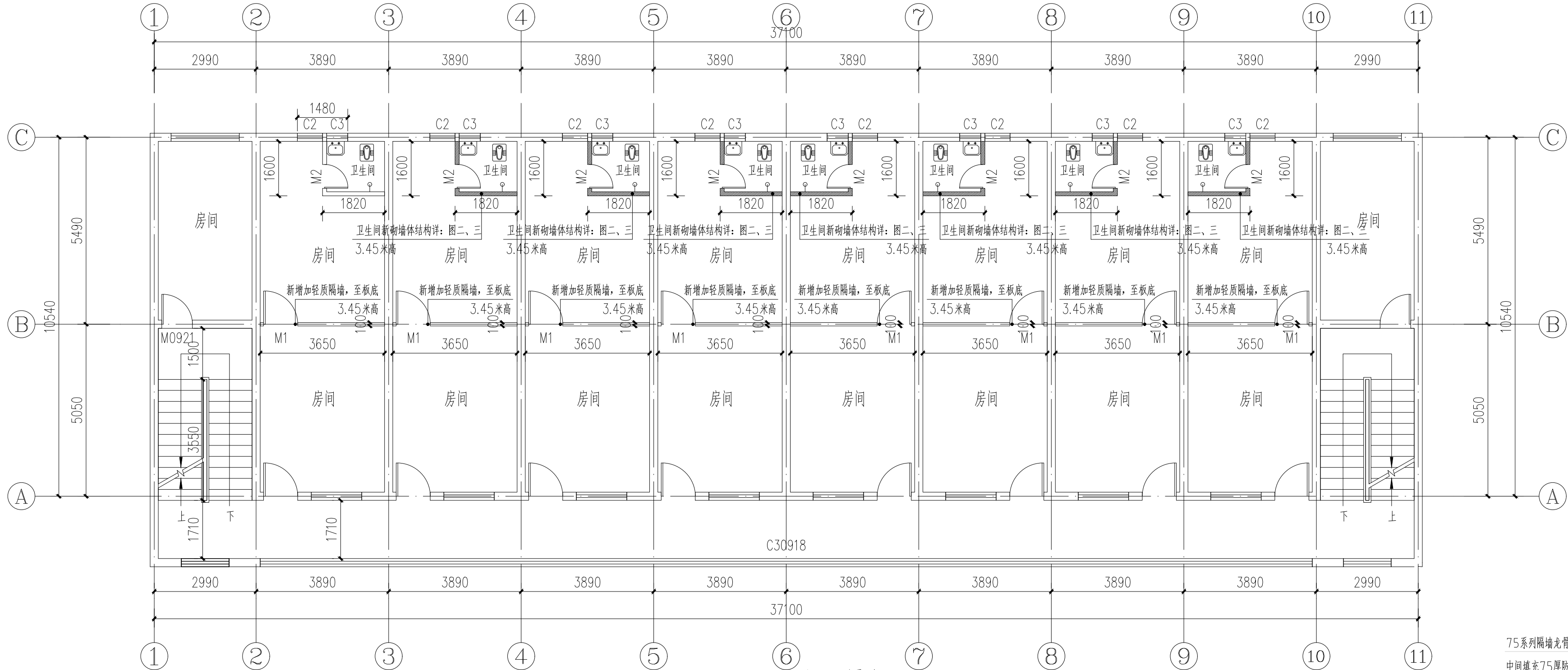
1号楼三层隔墙设计平面图 1:100
