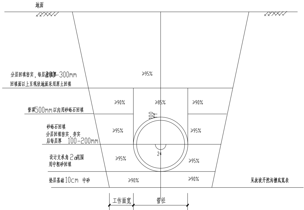
排水管沟槽开挖及回填断面图
