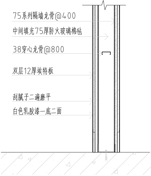
轻质隔墙大样图
