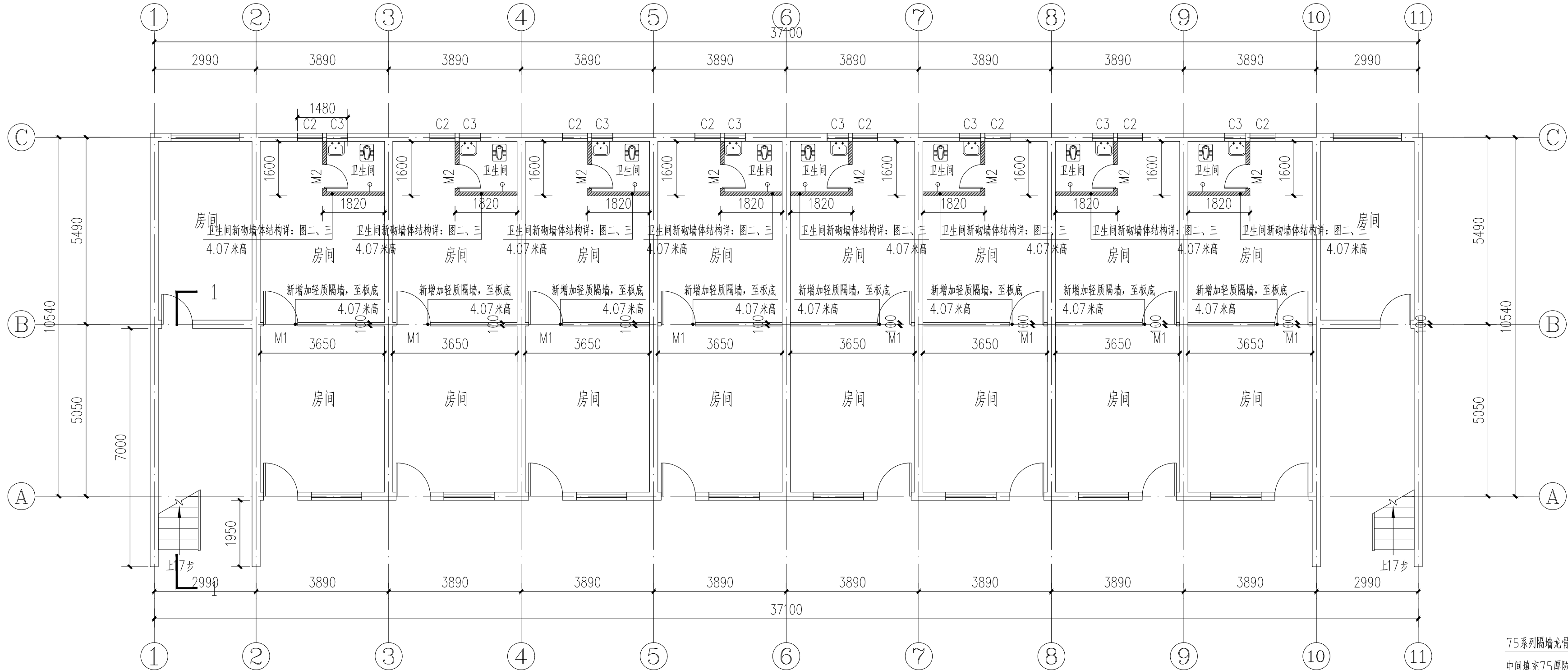
1号楼一层隔墙设计平面图 1:100
