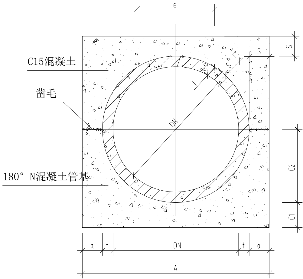
360° 混凝土满包加固管道基础断面图
