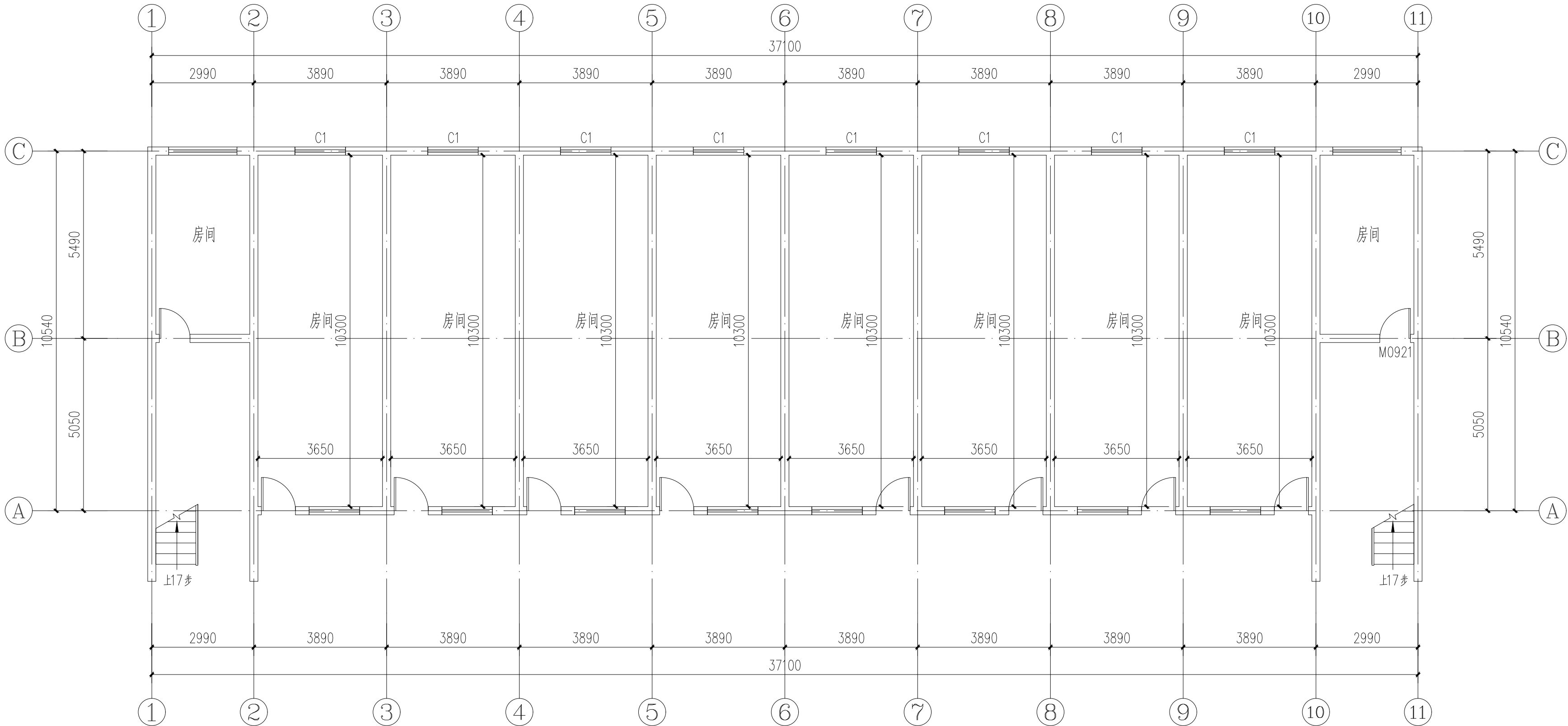
1号楼一层原始平面图 1:100
