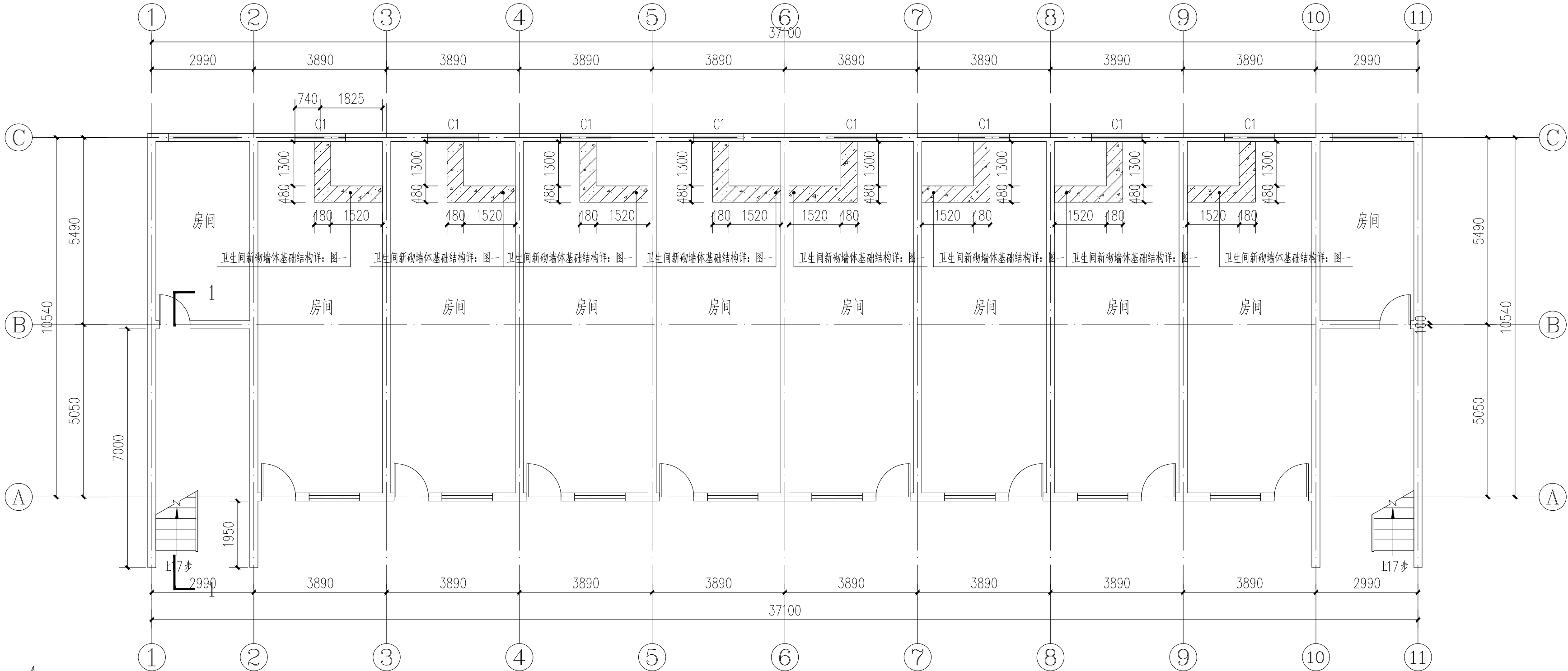
1号宿舍楼--一层至三层卫生间基础平面图 1:100
