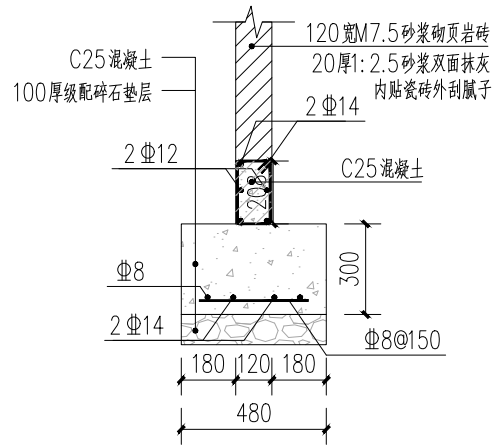
图一：一层卫生间隔墙基础图 1:20
