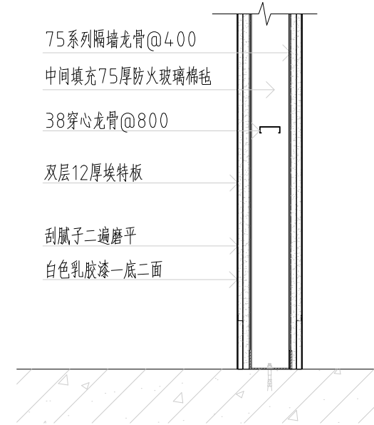
轻质隔墙大样图
