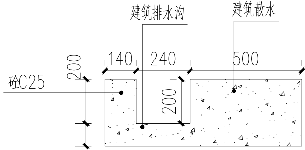
建筑排水沟建筑散水破除/修复大样图 1:20
