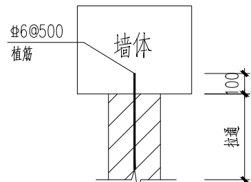
图二：墙拉筋详图
