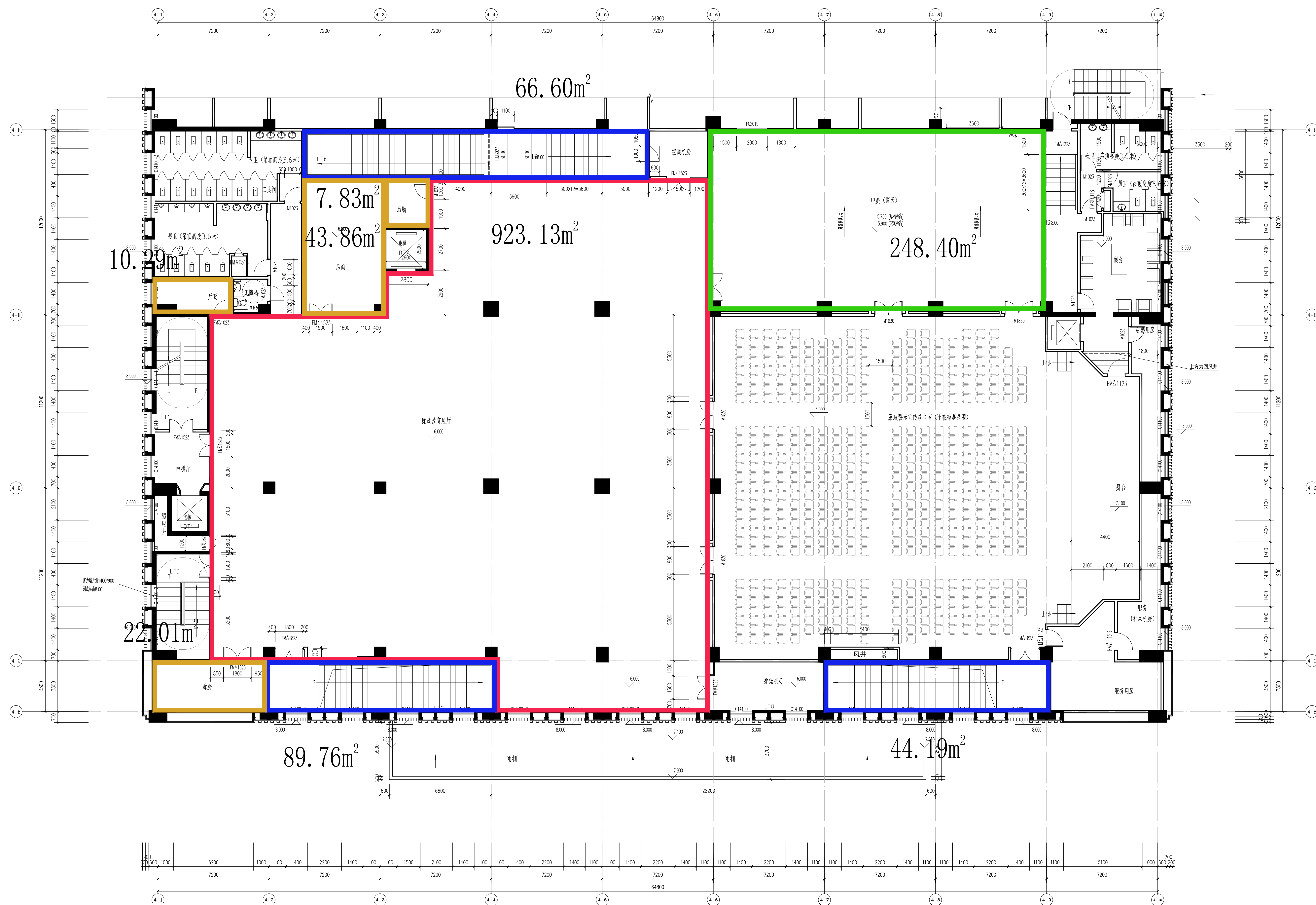
二层平面图
