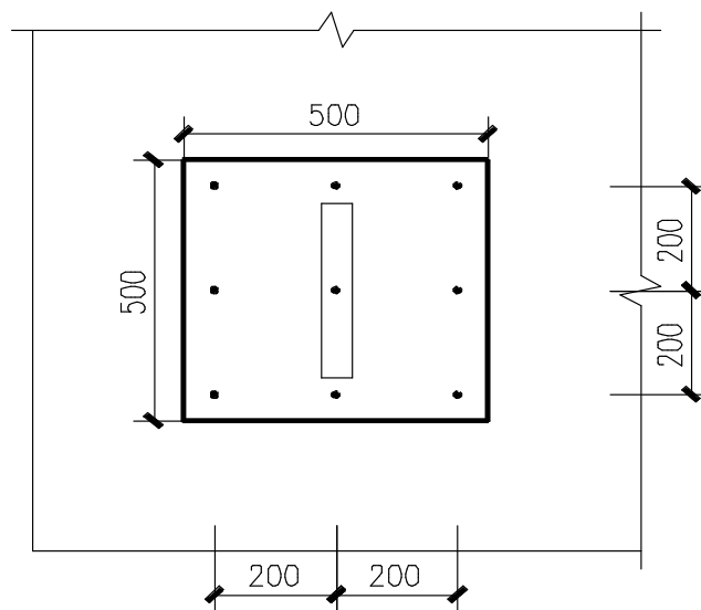
计算简图
