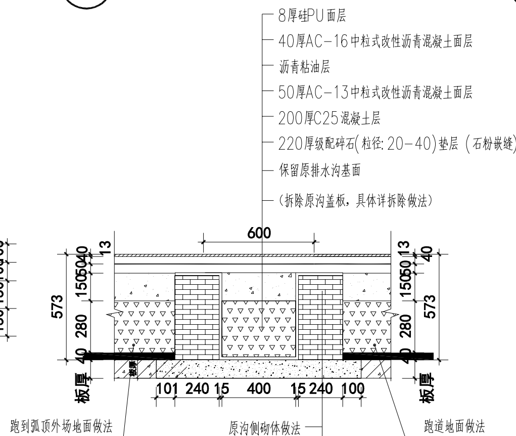
11 排水沟回填大样 1:20
