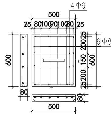
7 新建排水沟盖板配筋图 1:20
