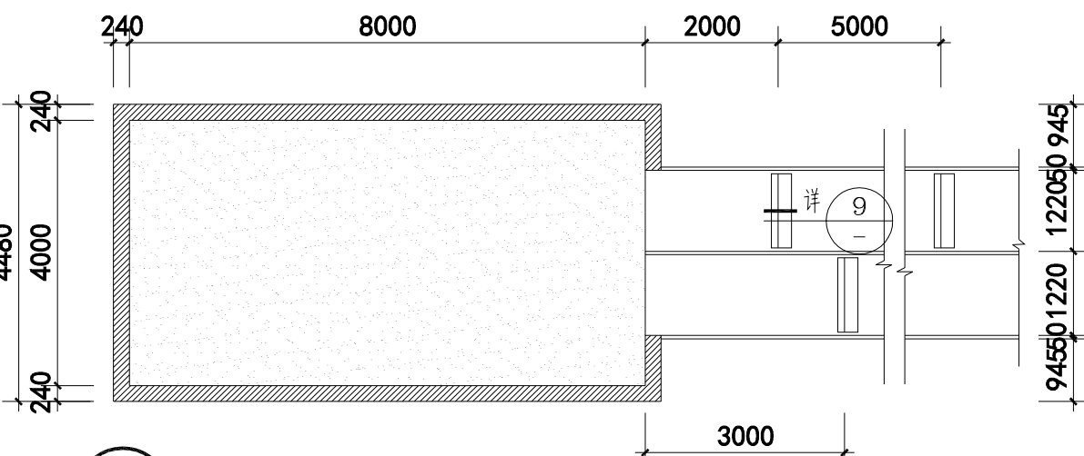
9 跳远砂坑平面详图 1:100
