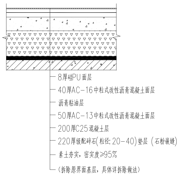
2 场地顶板外新做基层做法 1:20
