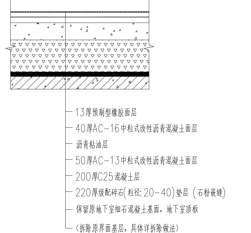
4 沙坑中间新做基层做法 1:20
