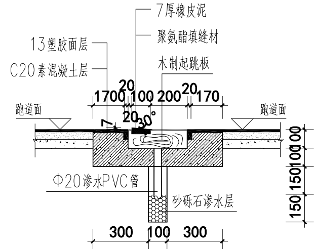
10 跳远起跳板大样 1:20
