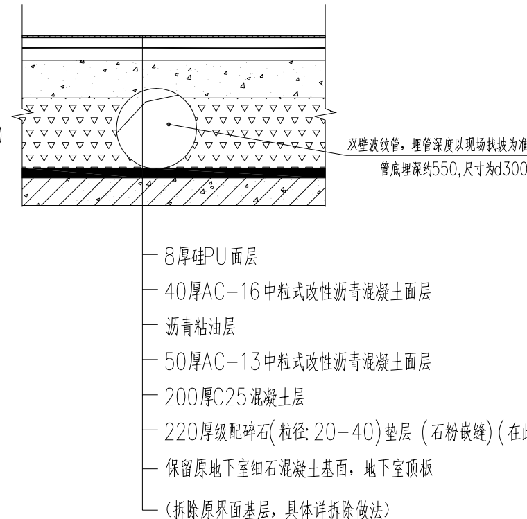
12 排水沟埋管大样 1:20
