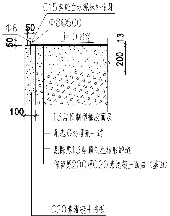
1 跑道基础断面 1:20
