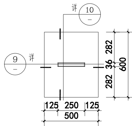
6 新建排水沟盖板平面图 1:20
