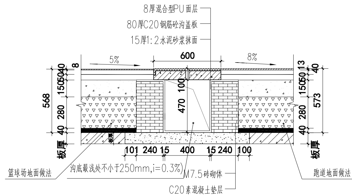
5 新建排水沟基础断面 1:20
