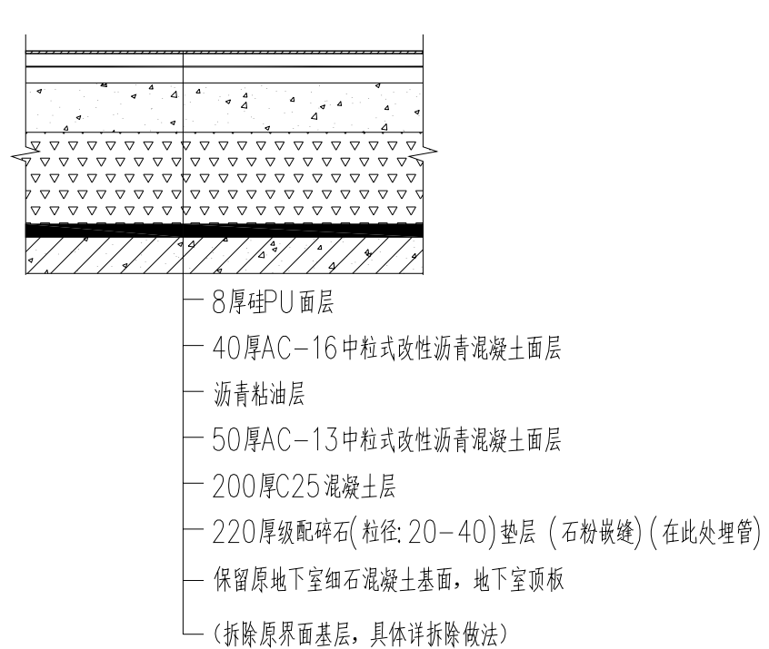
3 场地顶板内新做基层做法 1:20
