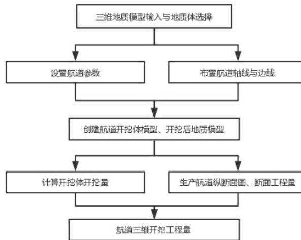
航道三维开挖模型建模流程图
