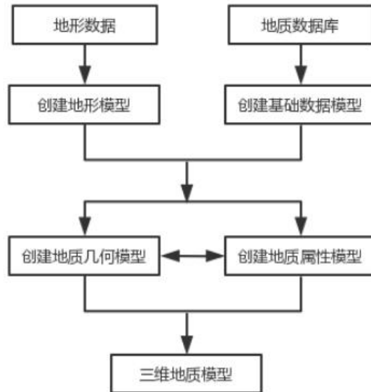
三维地质模型建模流程图
