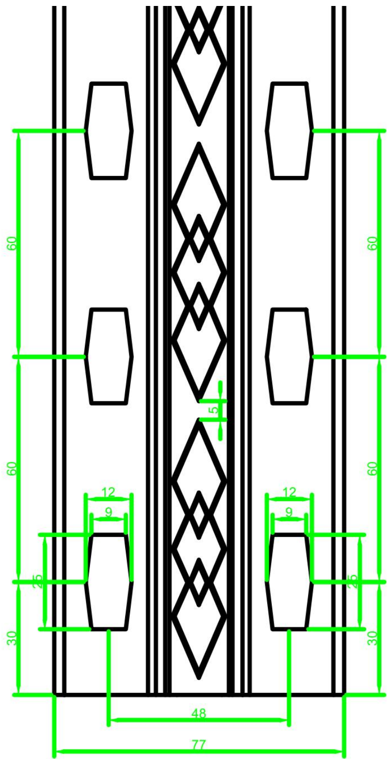
立柱正面图
