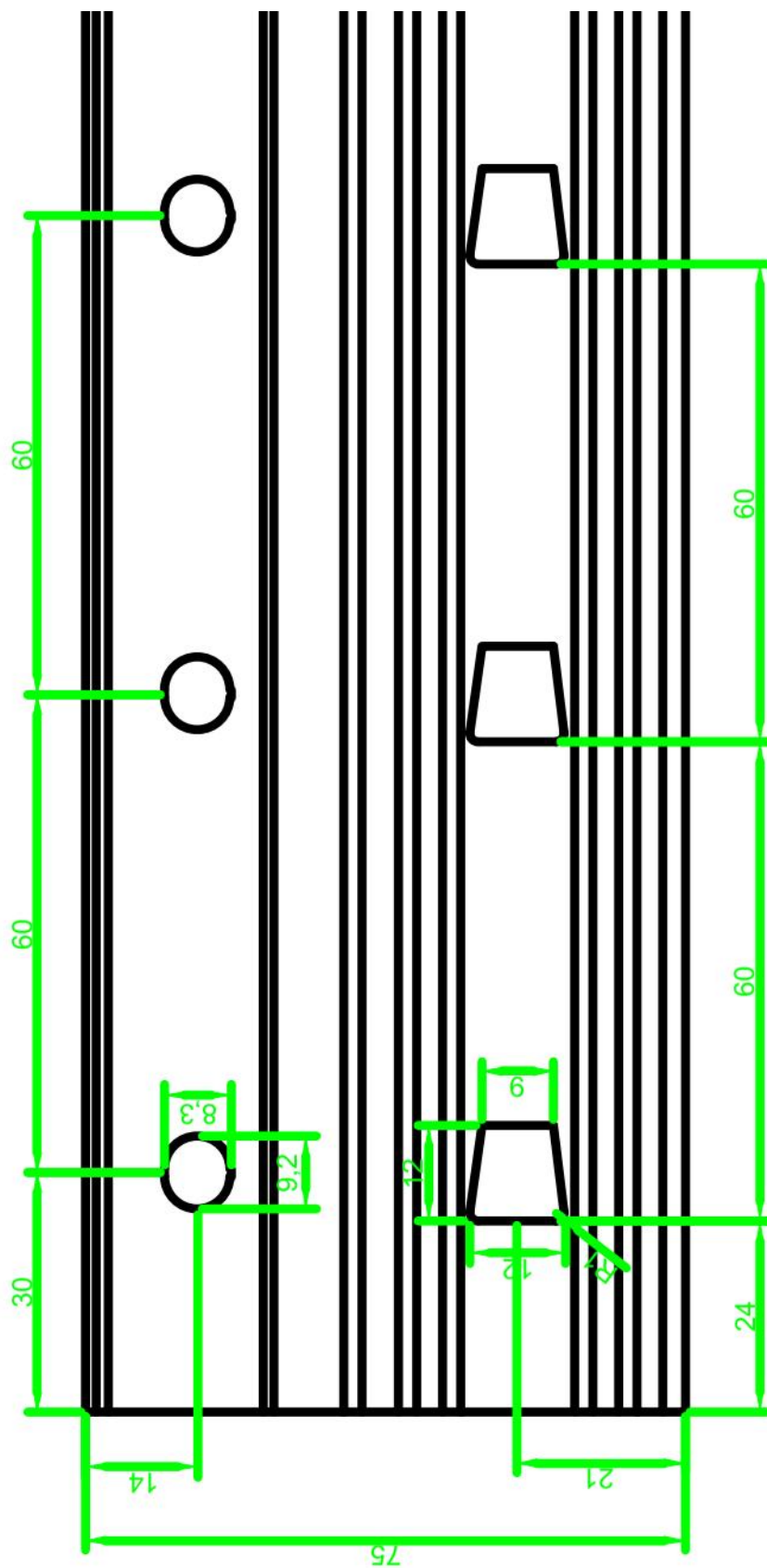
立柱侧面图
