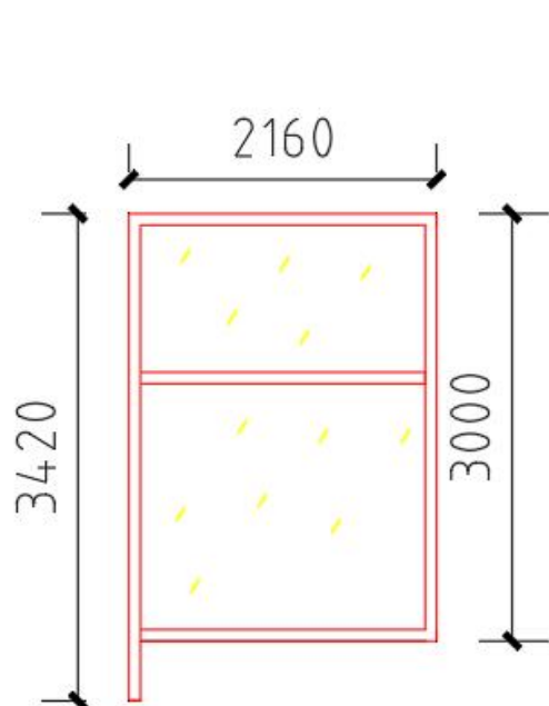
戒毒所玻璃隔断尺寸图
