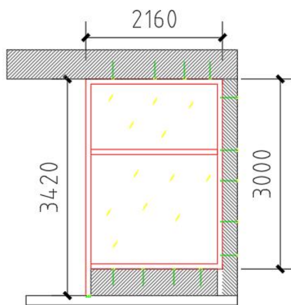
戒毒所玻璃隔断安装完尺寸图
