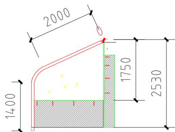
一看、二看玻璃隔断安装完尺寸图
