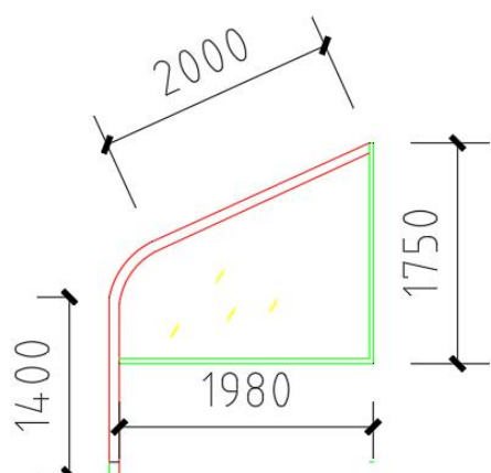
一看、二看玻璃隔断尺寸图
