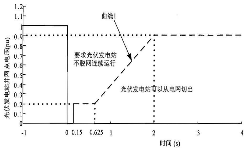
图 4.2.3-1 储能变流器低电压耐受能力要求
