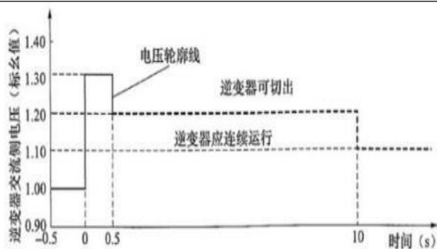
图 4.2.3-2 自动无功响应
